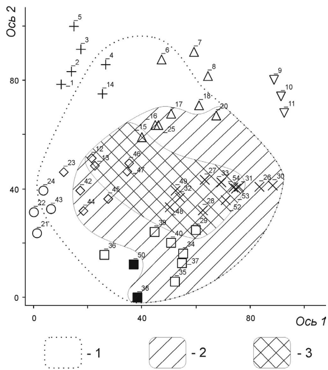
Рис. 1. Фитоценотический ареал (1), ареал с высокой встречаемостью (2) и фитоценотический оптимум (3) Carex lasiocarpa Названия ассоциаций (1–54) см. в табл. 3
