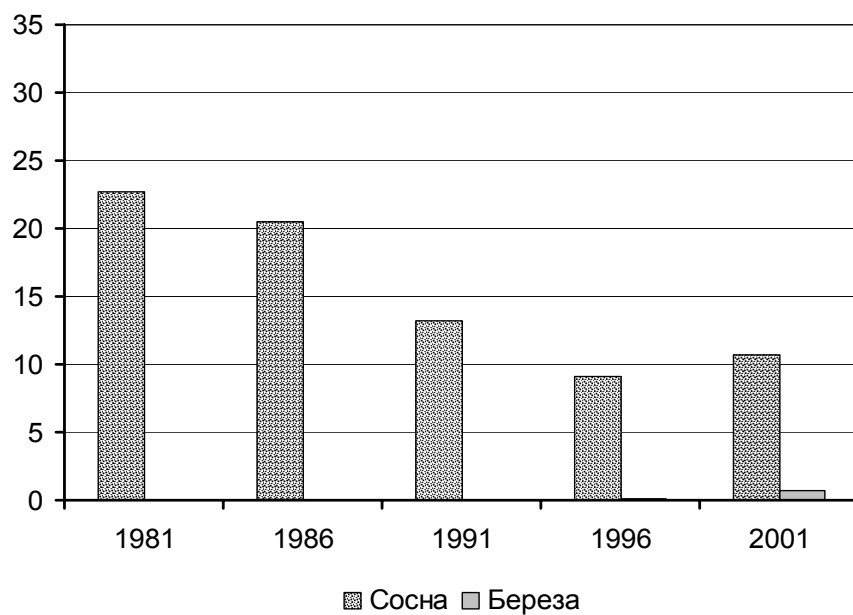
Рис. 2. Динамика древостоя сосняка сфагнового за 1981—2001 гг.
