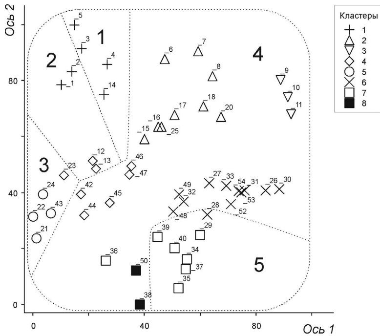
Рис. 5. Сопоставление групп ассоциаций тополого-экологической классификации и классов эколого-флористической классификации Классы: 1 – Oxycocco-Sphagnetea ; 2 – Vaccinietea uliginosa ; 3 – Alnetea glutinosae ; 4 – Scheuchzerio-Caricetea nigrae ; 5 – Phragmiti-Magnocaricet Названия ассоциаций см. в табл. 3
