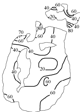
Рис. 2.10. Распределение фосфатов на поверхности Аральского моря (1961–1965, 1971–1975 и 1981–1985 гг. по: Гидрометеорология ..., 1990; 1992 г. по: Лю Хун, 1993), мг/л.
