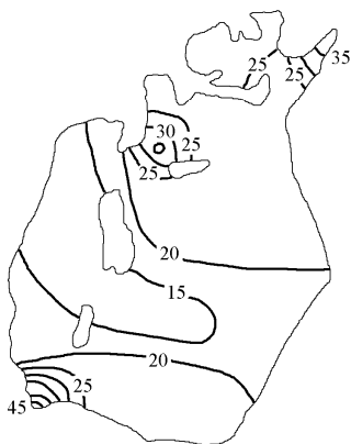
Рис. 2.10. Распределение фосфатов на поверхности Аральского моря (1961–1965, 1971–1975 и 1981–1985 гг. по: Гидрометеорология ..., 1990; 1992 г. по: Лю Хун, 1993), мг/л.
