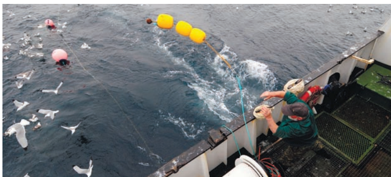
Рис. 9. Начало постановки стримерной линии
