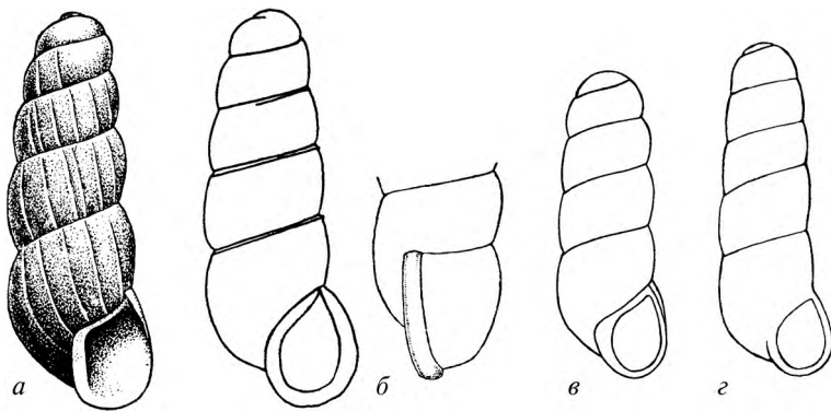
Рис. 306. Раковины видов Aciculidae:
