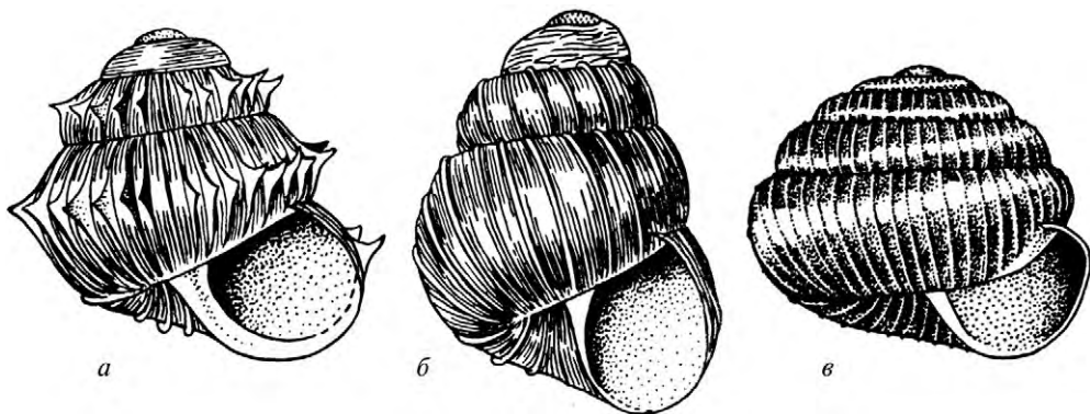
Рис. 45. Раковины видов Acanthinulinae (по Шилейко, 1984):
