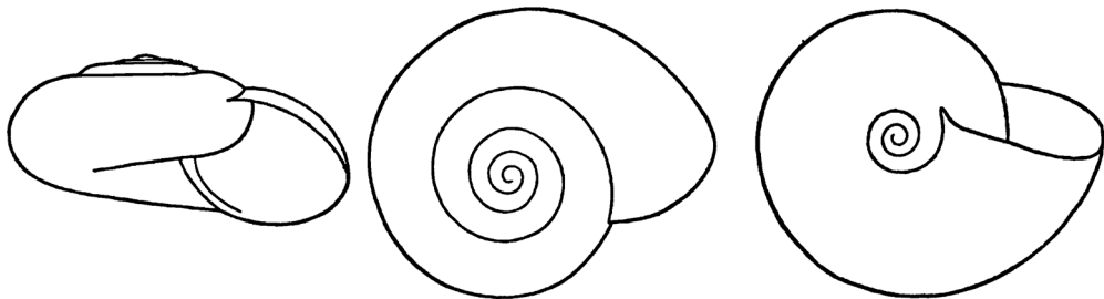
Рис. 114. Раковина Aegopinella minor (по Riedel, 1966)
