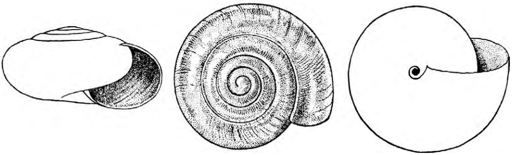
Рис. 104. Раковина Vitrea crystallina (по Лихарев, Раммельмейер, 1952)
