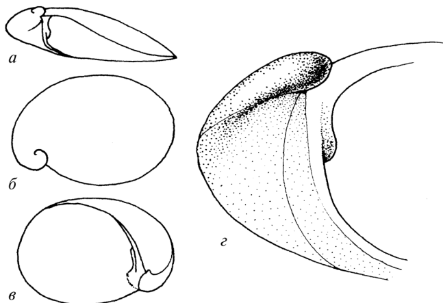
Рис. 153. Раковина Carpathica calophana (по Шилейко, 1986а):
