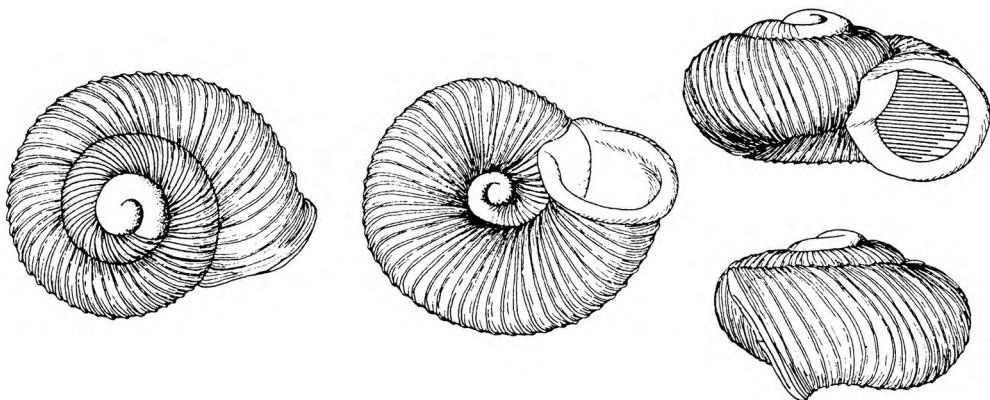
Рис. 48. Раковина Vallonia enniensis (по Gerber, 1996)
