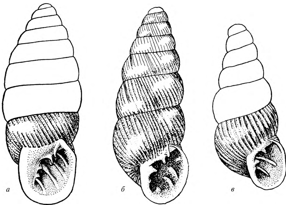
Рис. 60. Раковины видов Chondrinidae (по Шилейко, 1984): а — Granaria frumentum ; б — Chondrina arcadica caucasica ; в — Rupestrella rhodia
