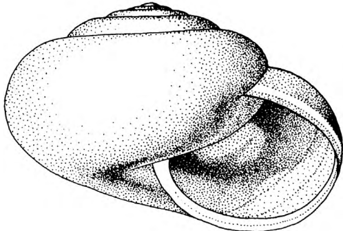
Рис. 292. Раковина Monacha fruticola (по Schileyko, 2006b)
