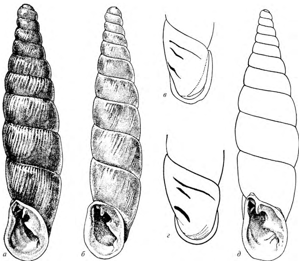
Рис. 80. Раковины видов Cochlodina (по Лихарев, 1962): a — C. orthostoma ; б, в — C. cerata ; г, д — C. laminata
