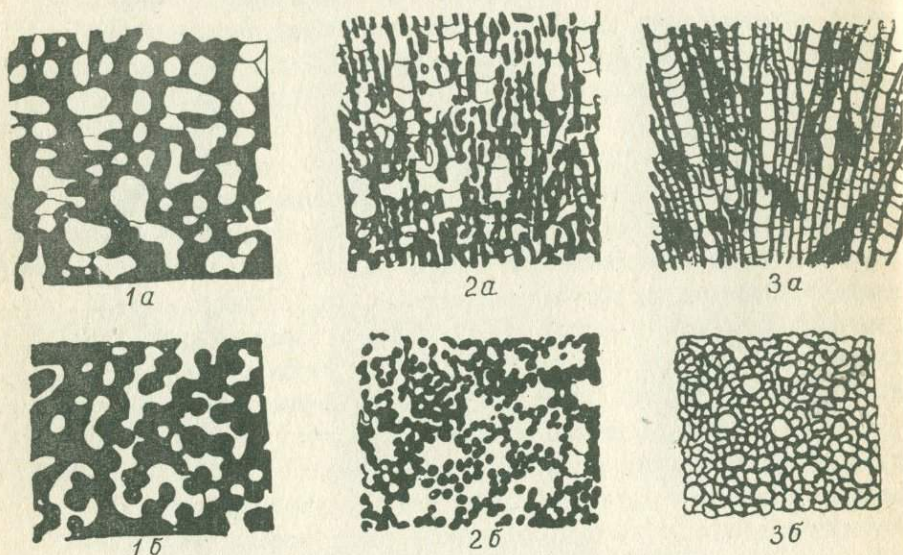
Рис.7. Зооидные трубки у строматопорид.
