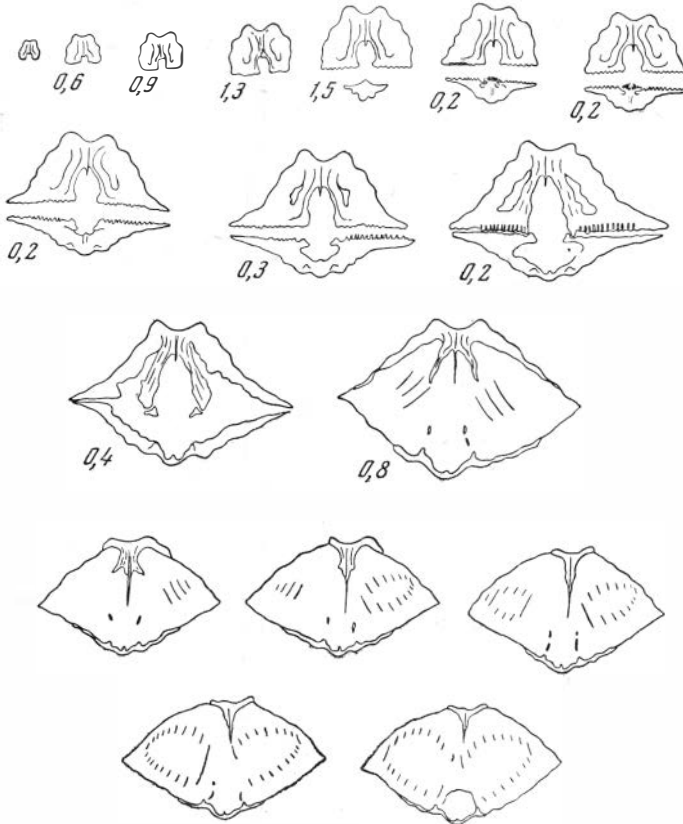
Рис. 46. Серия поперечных срезов двух экземпляров Orientospira pinguis sp. nov., р. Россоха (Булун), норийский ярус
