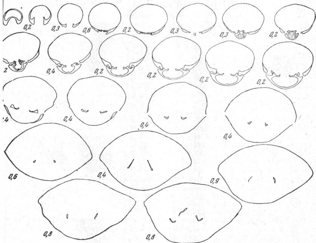
Рис. 61. Серия поперечных срезов раковины Lobothyris tuchkovi sp. nov., р. Визуальная, норийско-рэтские отложения
