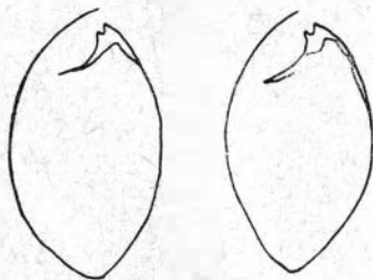
Рис. 18. Продольные срезы раковины Piarorhynchia formalis sp. nov., р. Русская, норвежско-рэтские отложения
