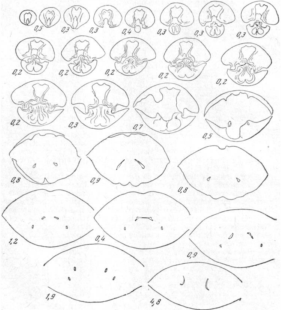
Рис. 62. Серия поперечных срезов раковины Kolymithyris kolymensis (Moiss.), р. Анманькаан, норийско-рэтские отложения
