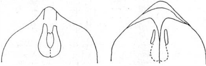
Рис. 36. Мускульные отпечатки Holcorhynchia borealis sp. nov., № 172/118; р. Алы-Юрях, карнийский ярус
