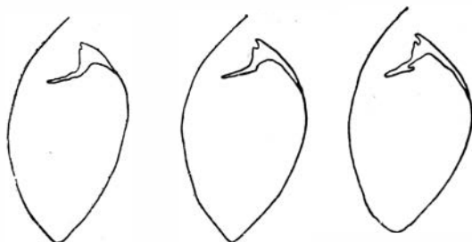
Рис. 10. Продольные срезы раковины Piarorhynchia yacutica sp. nov., р. Булкут, карнийский ярус
