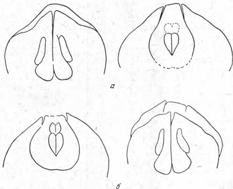
Рис. 16. Мускульные отпечатки Piarorhynchia diva sp. nov.
