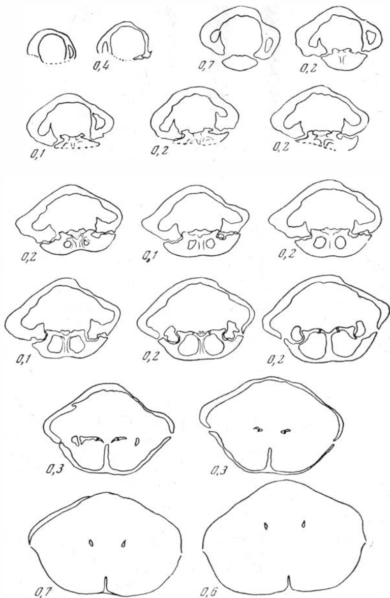
Рис. 41. Серия поперечных срезов раковины Maxillirhynchia sp., р. Анманьикан, норийско-рэтские отложения
