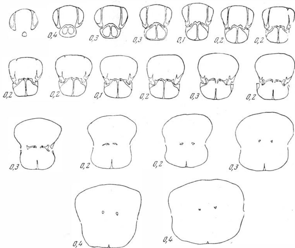
Рис. 25. Серия поперечных срезов раковины Sinuplicorhynchia kegalensis sp. nov., р. Кегали, карнийский ярус
