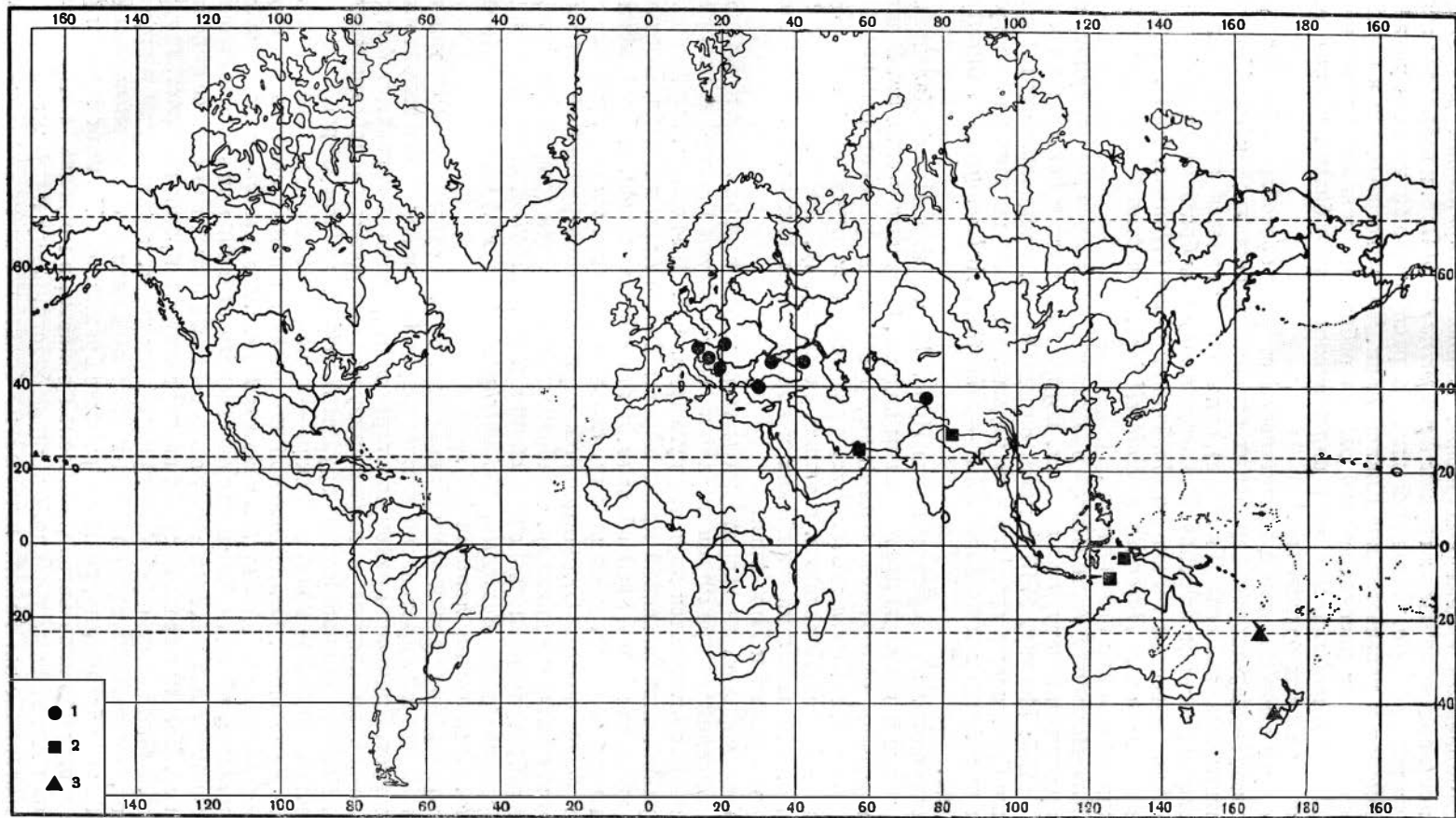
Рис. 66. Схема палеозоогеографического районирования южных морей в норийском и рэтском веках по брахиоподам: 1 — альпийская подобласть; 2 — индийская подобласть; 3 — австралийская подобласть
