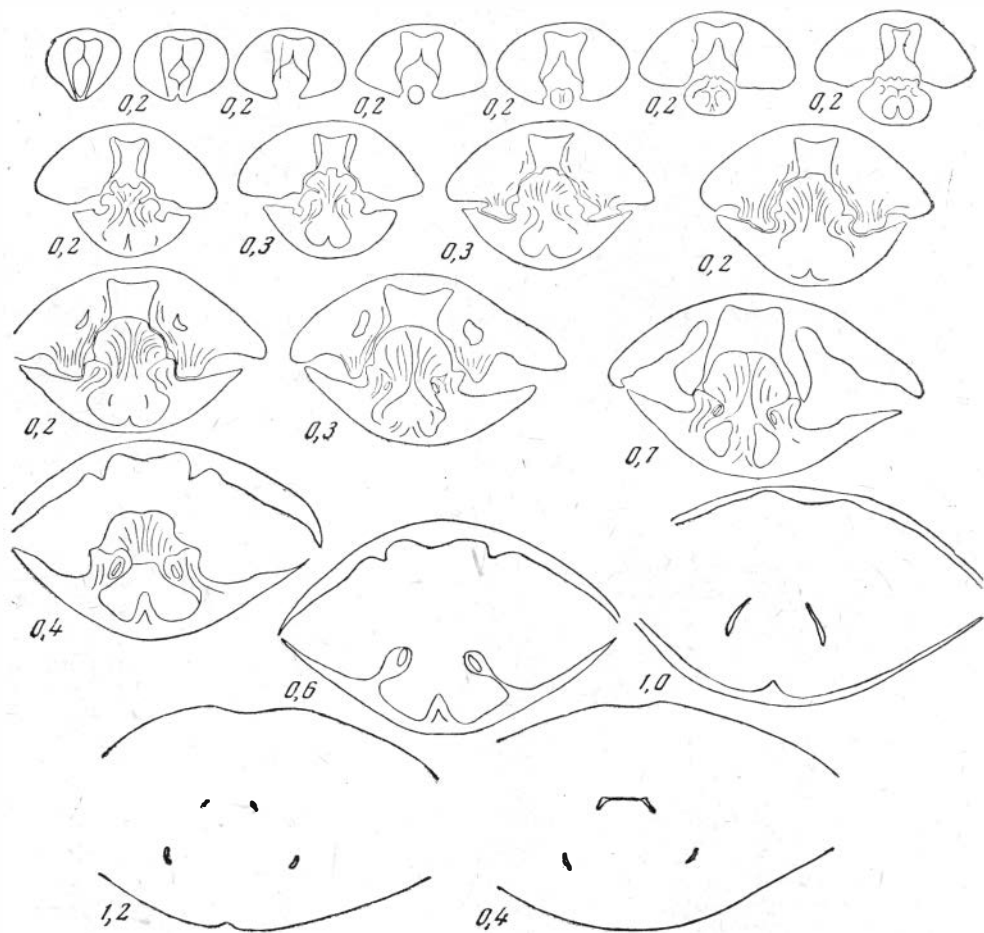
Рис. 63. Серия поперечных срезов раковины Kolymithyris orotshensis sp. nov., р. Россоха (Булун), карнийский ярус
