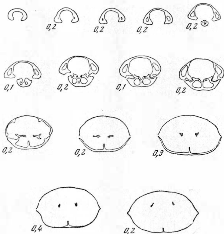
Рис. 38. Серия поперечных срезов раковины Holcorhynchia gizhigensis sp. nov. (молодой экземпляр); р. М. Туромча, карнийский ярус
