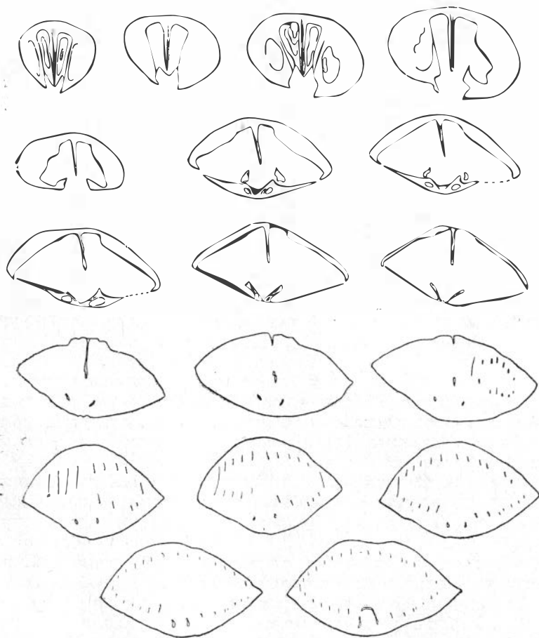
Рис. 50. Серия поперечных срезов раковины Viligella rotunda (Tuchkov), р. Авманныкан, норийско-рэтские отложения
