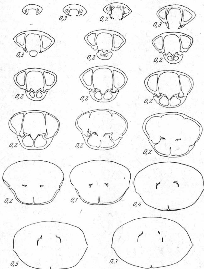
Рис. 7. Серия поперечных срезов раковины Piarorhynchia atrita sp. nov., р. Русская, норийско-рэтские отложения
