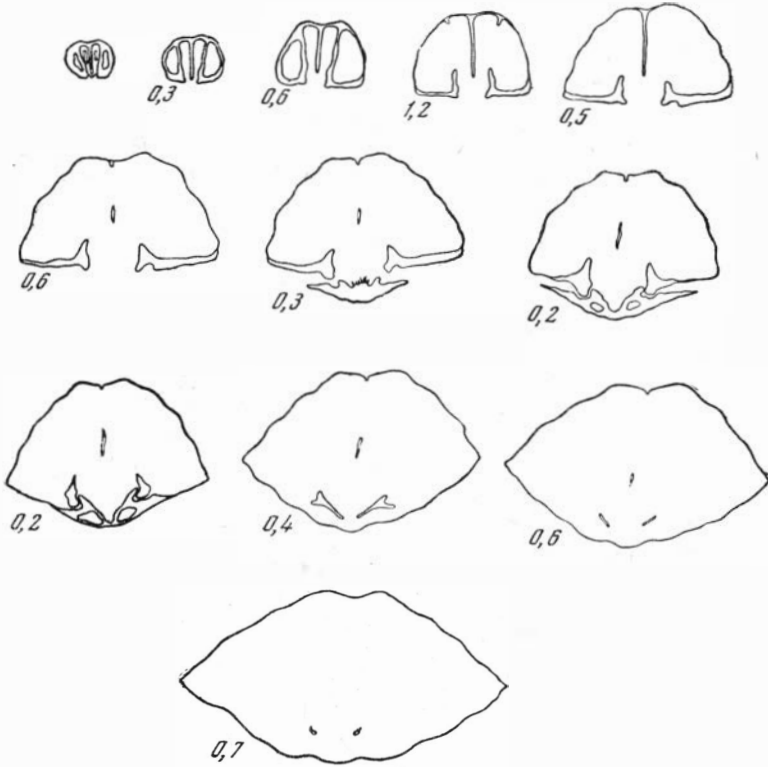
Рис. 53. Серия поперечных срезов раковины Spiriferina terekhovi sp. nov., р. Россоха (Булуц), карнийский ярус
