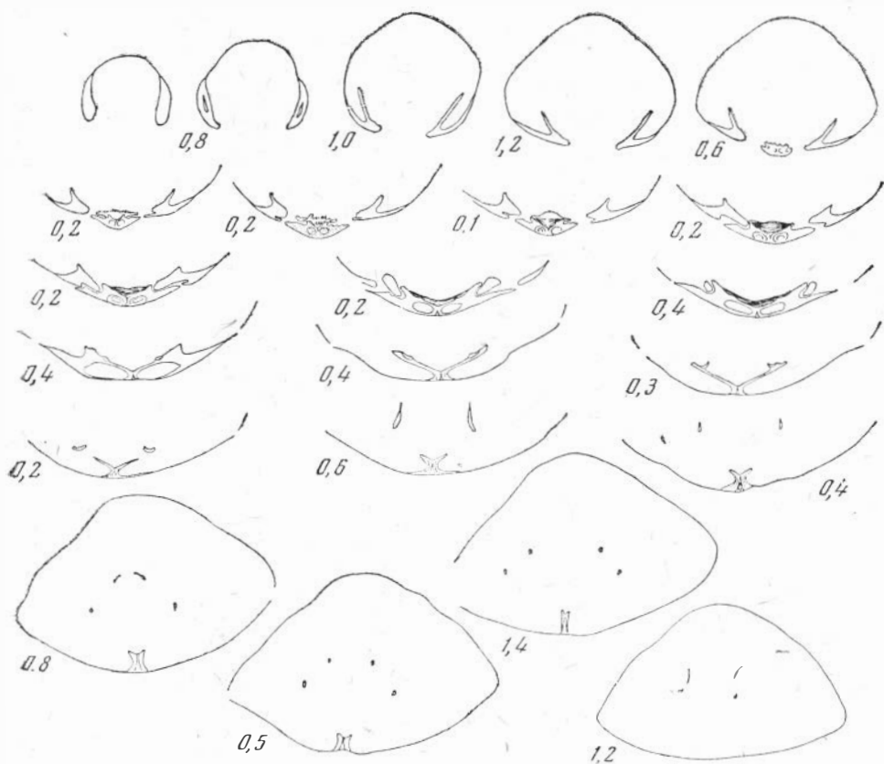
Рис. 65. Серия поперечных срезов раковины Aulacothyroides bulkutensis sp. nov., р. Булкут, карнийский ярус
