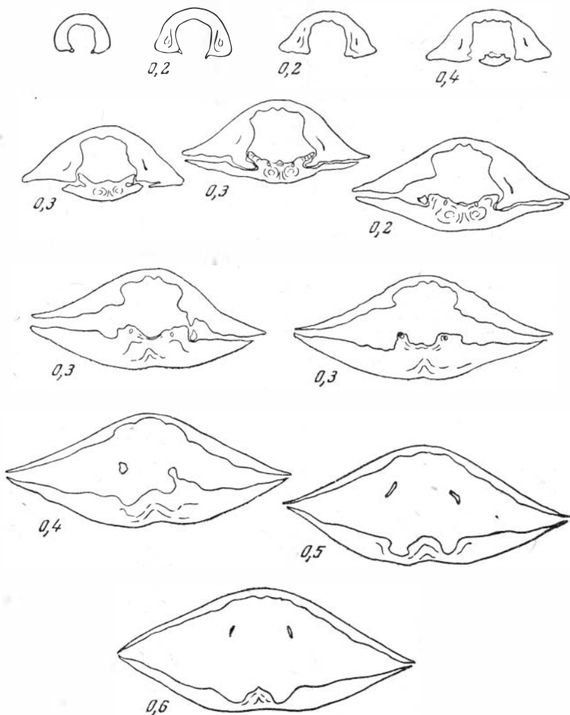
Рис. 31. Серия поперечных срезов раковины Norella tibetica Bitt., р. М. Туромча, карнийский ярус
