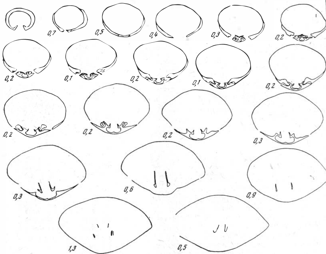
Рис. 60. Серия поперечных срезов раковины Lobothyris rossochae sp. nov., р. Россоха (Булуң), карнийский ярус
