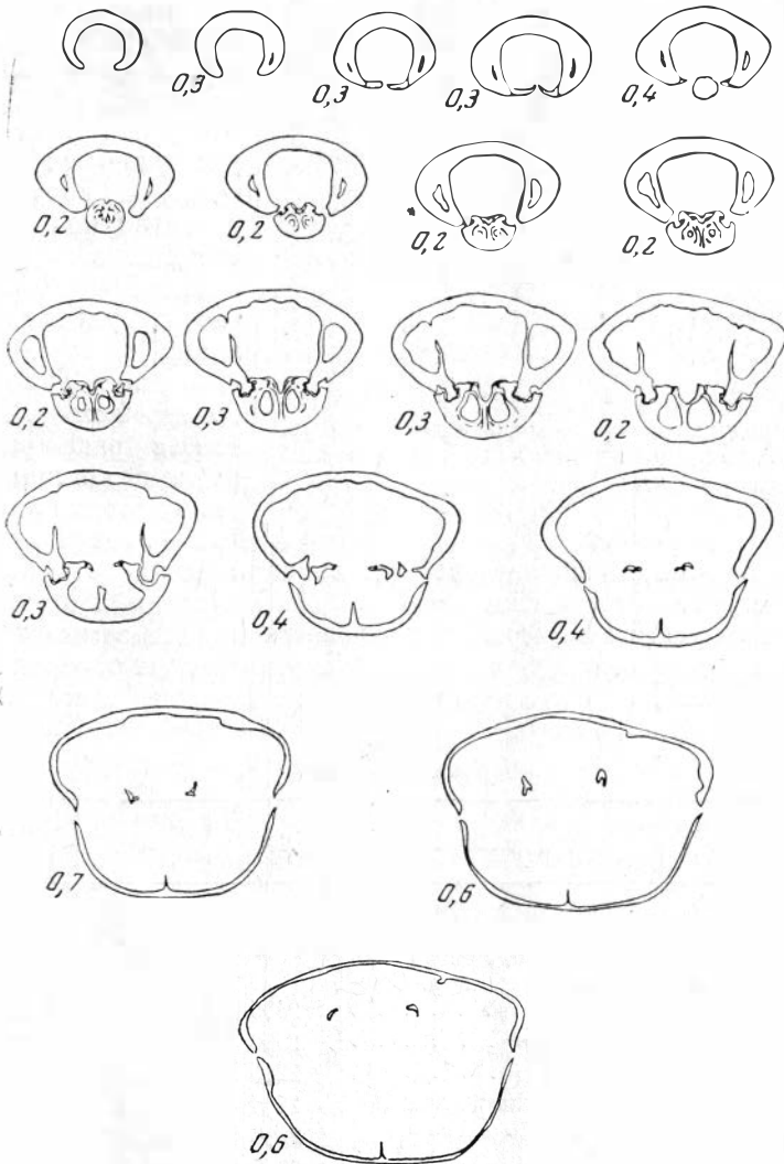
Рис. 14. Серия поперечных срезов раковины Piatorrhynchia diva sp. nov., р. Русская, норийско-рэтские отложения
