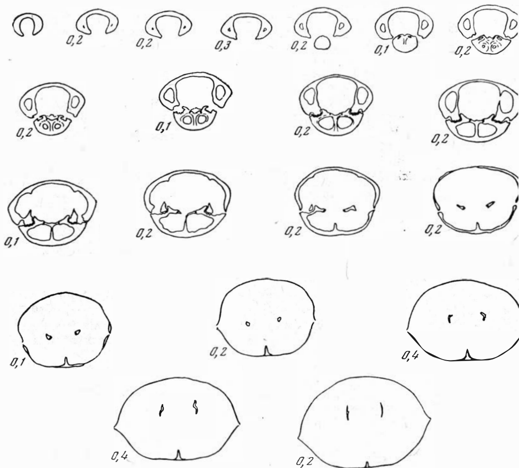
Рис. 12. Серия поперечных срезов раковины Piarorhynchia trinodosiformis sp. nov., р. Сейкмимян, карнийский ярус
