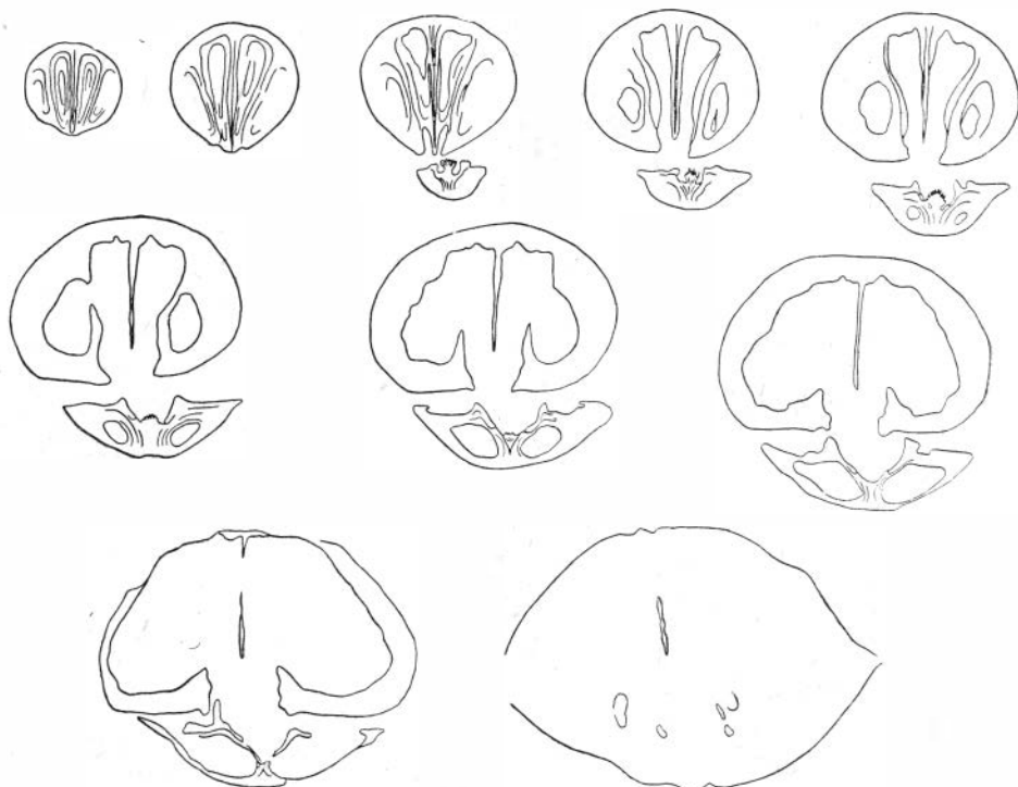
Рис. 51. Серия поперечных срезов раковины Viligella plicata sp. nov., р. Анманшкван, норийско-рэтские отложения
