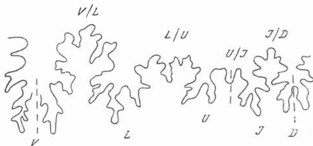
Рис. 1. Терминология элементов лопастной линии ( Porpoceras polare Frebold).
