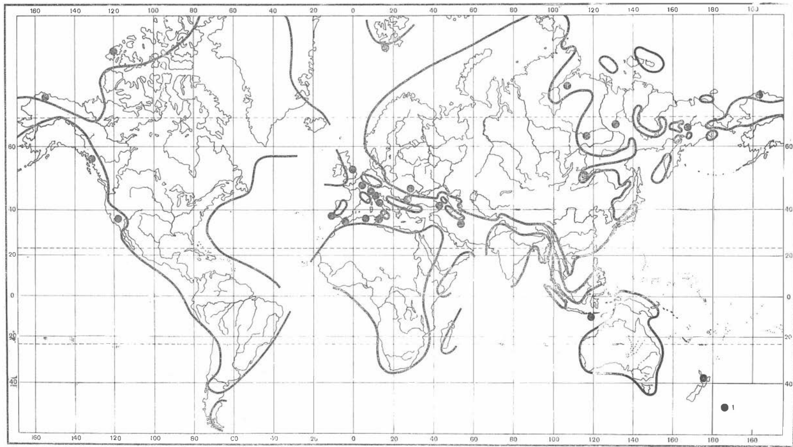
Рис. 27. Схема географического распространения среднетатарского рода Dactylioceras (1)
