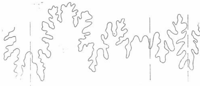
Рис. 11. Dactylioceras aff. stresherense Sapunov. Лопастная линия при Ш=8 мм. Экз. № 312—83, ×5,5
