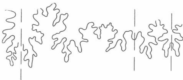
Рис. 21. Porpoceras polare (Friebold). Лопастная линия при D=14 мм, Ш=9 мм, V=4 мм. Экз. № 312—199, \times 5
