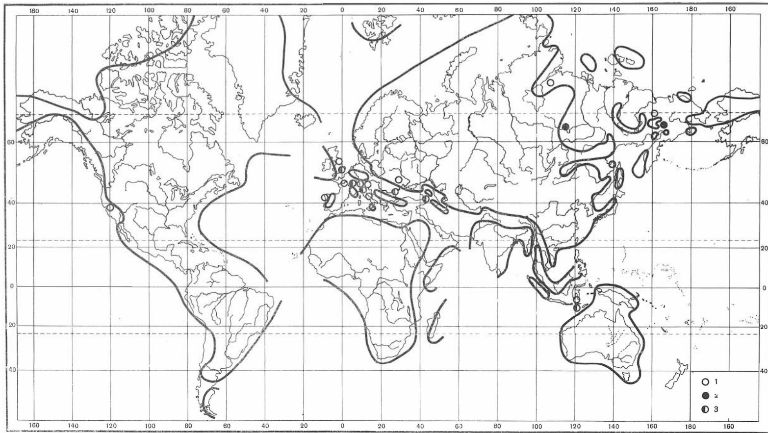
Рис. 28. Схема географического распространения среднетюрских родов:
