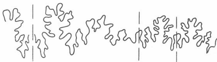
Рис. 19. Kedonoceras asperum sp. nov. Лопастная линия при Ш=8 мм. Экз. № 312—150, ×5
