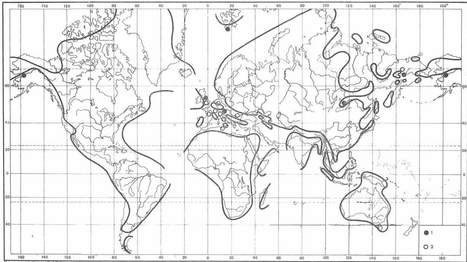
Рис. 29. Схема географического распространения верхнетриасовых родов
