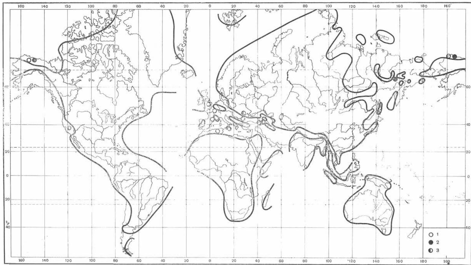
Рис. 26. Схема географического распространения нижнетроих родов 1 — Orthodactylites ; 2 — Kedonoceras ; 3 — Nodicoeloceras
