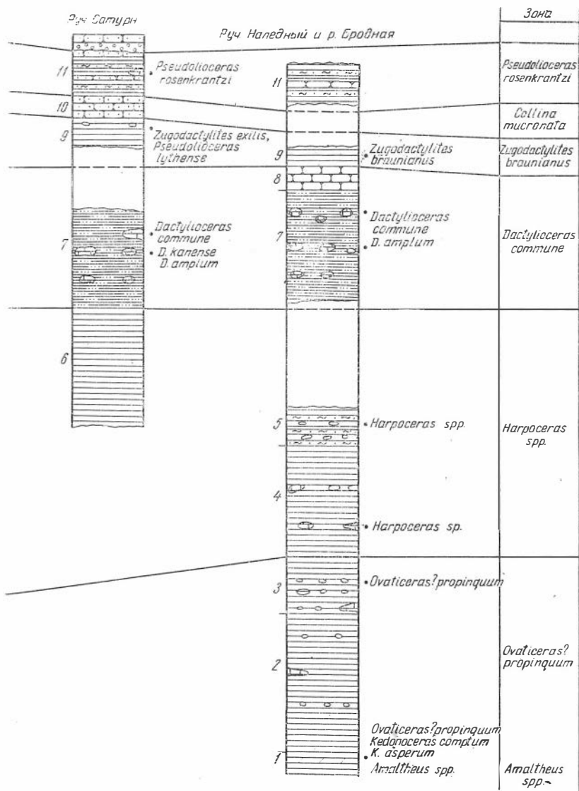
ний на Омолонском массиве 6 — известковые стяжения; 7 — мергели
