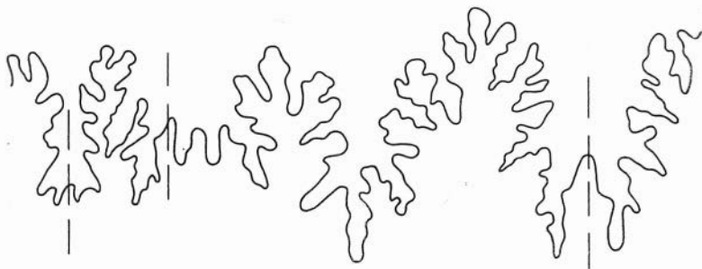
Рис. 12. Dactylioceras athleticum (Simpson). Лопастная линия при Ш=10 мм. Экз. № 312—198, \times 4
