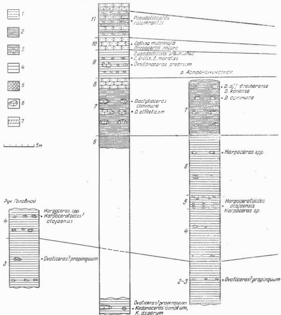
Рис. 23. Сопоставление разрезов тоарских отложений: 1—глины; 2—песчанистые глины; 3—алевролиты; 4—песчаники; 5—конгломаты;
