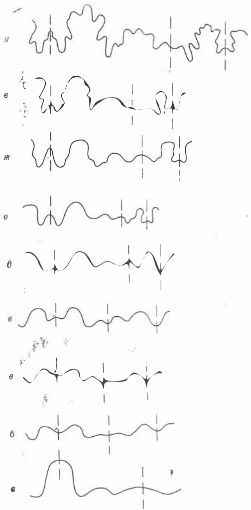
Рис. 20. Изменение лопастной линии в онтогенезе у Kedonoceras asperum sp. nov.
