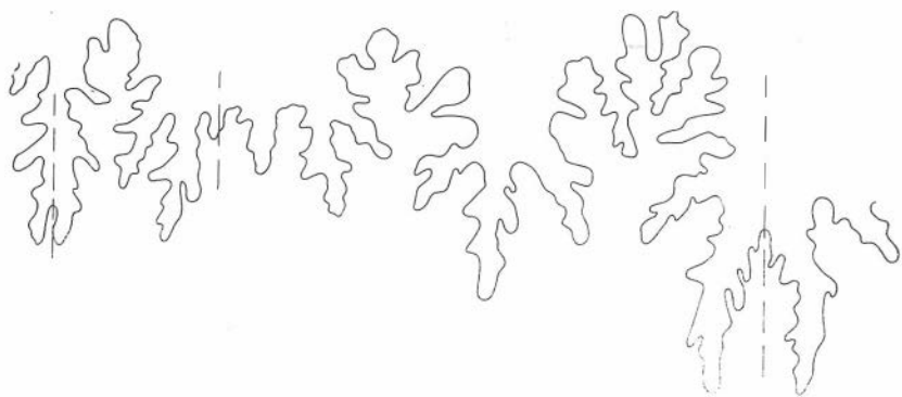
Рис. 10. Dactylioceras amplum sp. nov. Лопастная линия при Ш=13 мм. В=10 мм. Экз. № 312—70, \times 5,5
