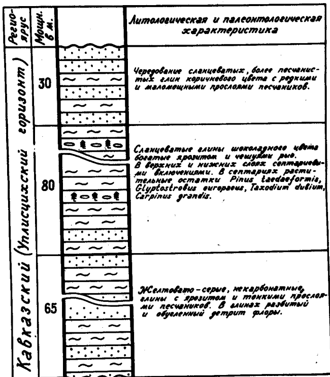
Рис.5. Стратиграфический разрез в окр. с.Цедиси
