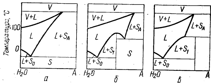
Рис. 9. Общий вид диаграмм состояния систем неорганическое вещество — вода с образованием:
