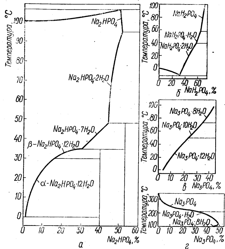
Рис. 24. Системы фосфаты натрия — вода:
