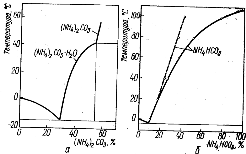
Рис. 12. Системы карбонат, гидрокарбонат аммония — вода (а, б).
