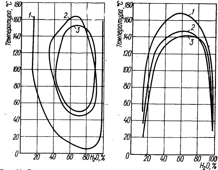
Рис. 33. Бинарные системы метилпиридины — вода:
