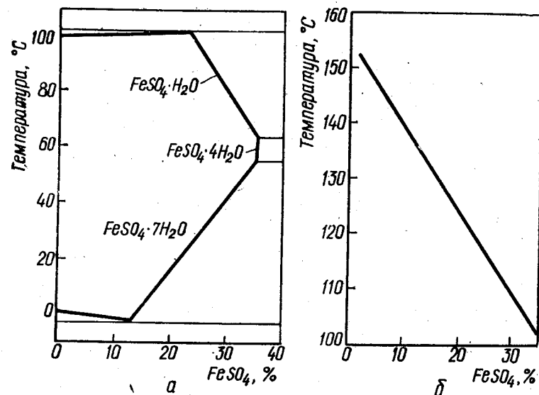
Рис. 22. Система \text{FeSO}_4\text{—H}_2\text{O} :
