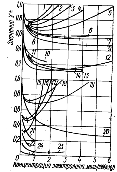
Рис. 39. Коэффициенты активности электролитов при 26 °C: 1 — HCl; 2 — LiCl; 3 — NaI; 4 — NaBr; 5 — NaCl; 6 — KCl; 7 — NH 4 Cl; 8 — NaF; 9 — CsCl; 10 — Na 2 CO 3 ; 11 — K 2 SO 4 ; 12 — H 2 SO 4 ; 13 — Na 2 SO 4 ; 14 — (NH 4 ) 2 SO 4 ; 15 — AlCl 3 ; 16 — MgCl 2 ; 17 — CaCl 2 ; 18 — KOH; 19 — NaOH; 20 — NaH 2 PO 4 ; 21 — Na 2 HPO 4 ; 22 — Na 3 PO 4 ; 23 — MgSO 4 ; 24 — Al 2 (SO 4 ) 3 .
