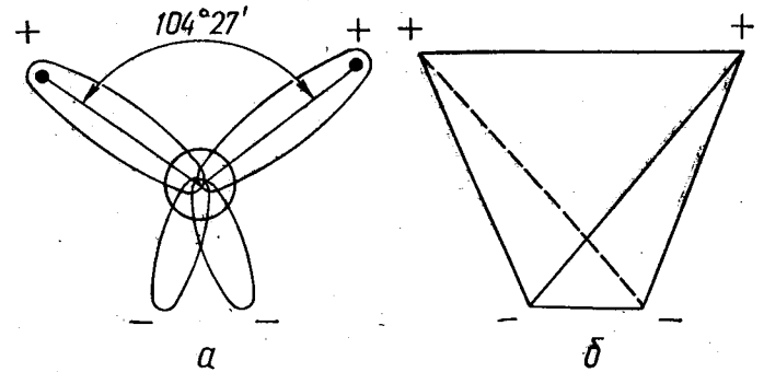
Рис. 6. Строение молекулы воды: а — структура электронного облака молекулы; б — расположение полюсов заряда.
