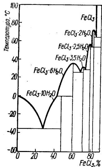
Рис. 21. Система \text{FeCl}_3\text{—H}_2\text{O} :
