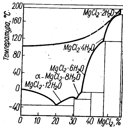
Рис. 17. Система \text{MgCl}_2\text{—H}_2\text{O} :
