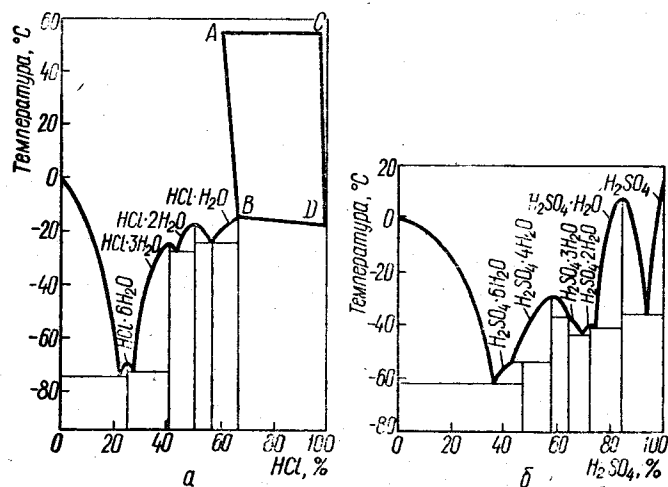
Рис. 29. Системы \text{HCl}-\text{H}_2\text{O} (а) и \text{H}_2\text{SO}_4-\text{H}_2\text{O} (б):
