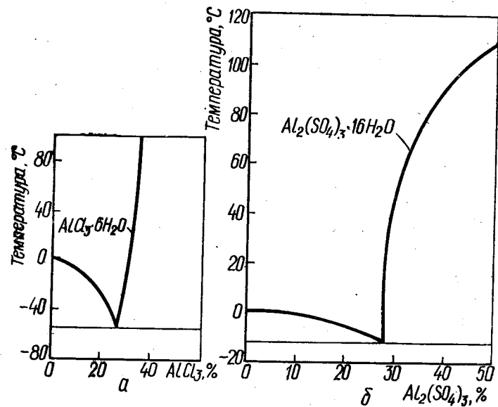
Рис. 20. Система \text{AlCl}_3\text{—H}_2\text{O} ( a ) и \text{Al}_2(\text{SO}_4)_3\text{—H}_2\text{O} ( b ):
