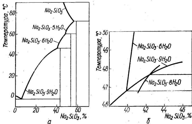
Рис. 25. Система \text{Na}_2\text{SiO}_3 - \text{H}_2\text{O} :
