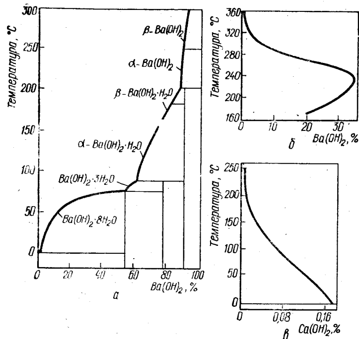
Рис. 31. Системы \text{Ba}(\text{OH})_2\text{—H}_2\text{O} (а, б) и \text{Ca}(\text{OH})_2\text{—H}_2\text{O} (в):
