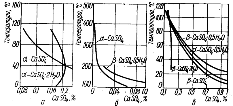
Рис. 18. Система \text{CaSO}_4\text{—H}_2\text{O} :
