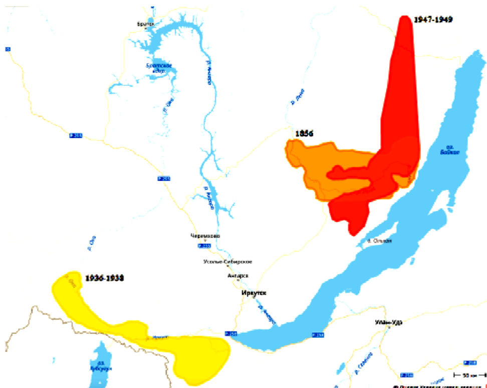
Рис. 8. Районы массового размножения серой лиственничной листовертки в Восточной Сибири (по Флорову, 1952)
