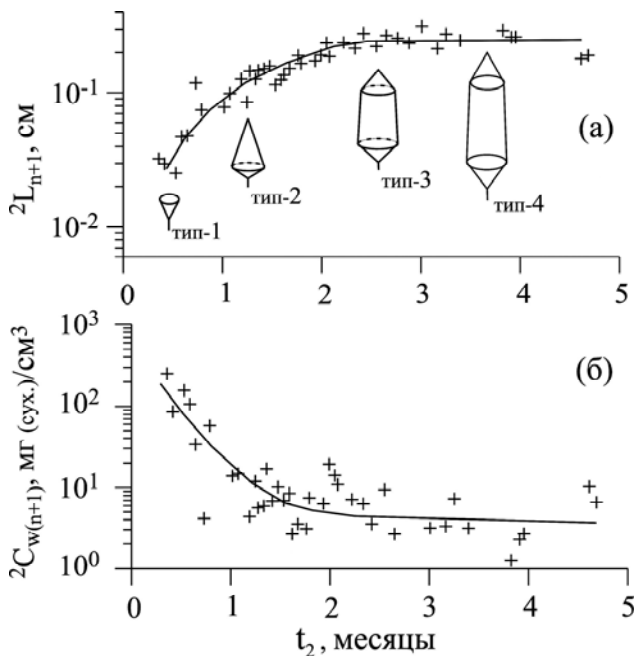
Рис. 5.8. Изменение характерной длины метаболического пути ( L_{n+1} , а) и объемной концентрации сухого вещества ( C_W , б) в субкрупном пространстве ветвей второго порядка Cystoseira crinita в их онтогенезе ( t_2 )
