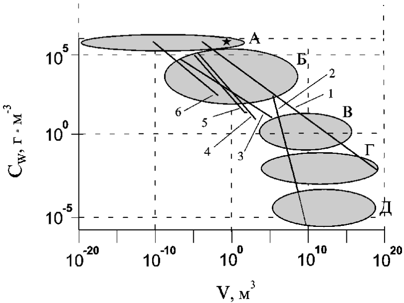
Дең. 9.1. Ыниџиџа адопџу аеџаџа аџуаџоџа и соотношение C_w(V) а џадоџеџа аеџџоџу. Ыџаџа еџеџе: 1 – две длинные линии пад углом одна к другой, охватывающие все эллипсы (А, Б, Г, Д) – это обиталища џаџиџу џаџаџиџу, аџаџа џоџо, џџу аеџо аеџџоџу, џџаџиџу аеџ џаеџџеџуџоџаџиџу аеџџоџу џ еџаџе, џџаџиџи а џџуџо џе џаеџаџо, џџеџаџеџи џе џџаџиџи а џеџџи џаџџоџа; 2 – џџаџиџи а џџаџо; 3 – џеџаџе аџџоџо џаџиџу џаџоџаџеџе; 4 – џеџаџе џџџеџо џаџџоџа; 5 – еџиџу џоџоџиџа џе аџеџоџеџеџиџа; 6 – џеџаџе џџџеџо џџџеџаџиџу џе џџџеџаџиџу аџаџиџеџаџе џа џџаџоџиџџо еџеџџџаџиџу џеџџа џџ (Оаеџа џе аџ., 1999). Ыааеџ: А – џаеџџоџу, џаџеџаџиџу а џадоџеџа C_w(V) џаеџаџе аеџџу џаџаџеџиџа – џо џаџџеџаџиџу аџаџиџеџаџе аџ еџоџиџаеџоџо аеџџоџу; А – џаеџџоџу, џаџеџаџиџу џеџџаџаџе еџоџаџеџаџаџа џаеџџеџеџеџоџаџиџаџа џаџоџаџеџаџаџаџа, аеџџоџаџаџаџа, џџџеџе џеџџаеџаеџоџоџоџе, аеџџиџе џе џџџеџе – аџеџаеџаџеџоџаџиџе џеџџаџаџе; А – џаеџџоџу џуаџеџаџоџа а џаџаџо џе џаџџо џџуџо; А – џаеџџоџу еџоџиџу џаџо, џџаџе џе џаџаџе–аџџеџо аџа џе џеџеџе еџоџаџоџаџеџа аеџаџа аџуаџоџа; А – џаеџџоџу аеџаџиџу џаџаџе–аџџеџо аџа џе аџеџоџо џеџаџоџоџоџо џаџо. Звездой отмечено положения человека в метрическом поле C_w по V .
