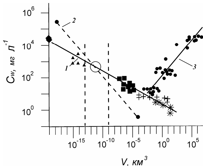
Рис. 8.5. Соотношение между геометрическим объёмом ( V_n, V_{n+1} ) водных биокосных объектов с концентрацией ( C_w ) суммы растворённых в воде органических веществ (РОВ) в их внутренней среде. Линия 1 слева направо: клеточный сок морских многоклеточных водорослей (♦), в крови рыб (▲), вода в прудах и мелких озёрах с обильной водной растительностью (■), вода на мелководьях Чёрного моря (+), вода в океанах (*). Штриховая линия 2 показывает соотношение между геометрическим объёмом и концентрацией взвешенного "живого вещества" организмов (ВОВ) в аналогичных водных объектах. Линия 3 – солёность воды в водоёмах разного объёма.
