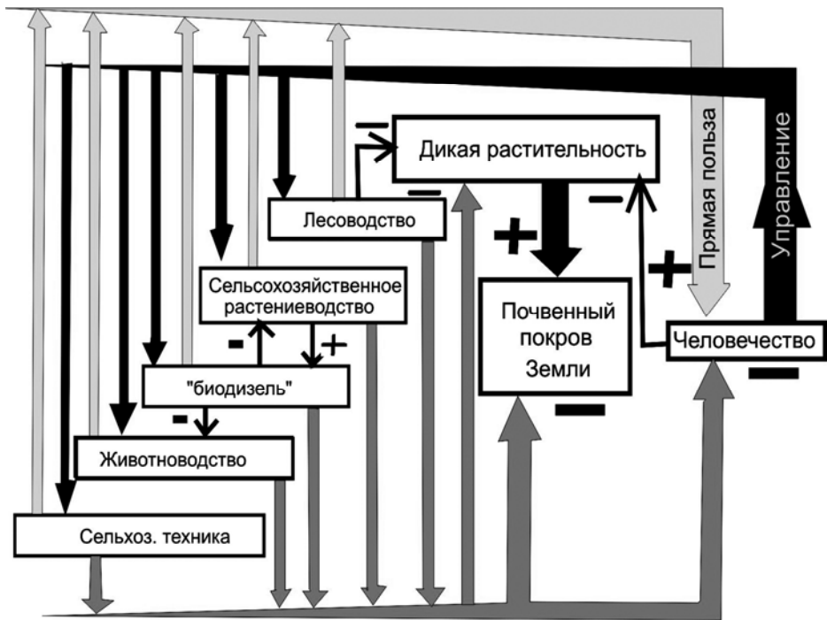
Рис. 1.4 Блок-схема главных природопользовательных связей между человечеством и остальной биосферой. Назовем три группы положительных (плюсы) и отрицательных (минусы) связей между человечеством и отдельными природными и рукотворными блоками: 1) прямая польза от рукотворных блоков, 2) людское управление отдельными блоками и 3) отрицательное, в основном отдаленное (отложенное) влияние рукотворных блоков на почвенный покров и человечество. Жирным контуром выделены главные жизнеопределяющие блоки. Главным хранителем почв и почвенного плодородия является дикая травянистая растительность, испытывающая на себе мощное отрицательное влияние человечества. Культурная травянистая растительность может оказывать положительное влияние на почвы лишь при определенных условиях, которые выдерживаются редко.
