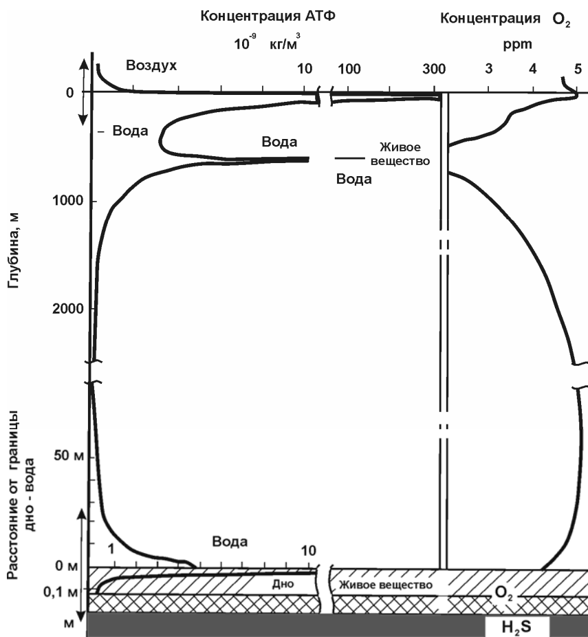
Рис. 8.12. Схема вертикального околосредового распределения кислорода, ATF и сероводорода в Атлантическом океане. Уместно сравнить эту схему и схему распределения структур в живой клетке (рис. 8.10.). Из: Lebedev et al., 1989.
