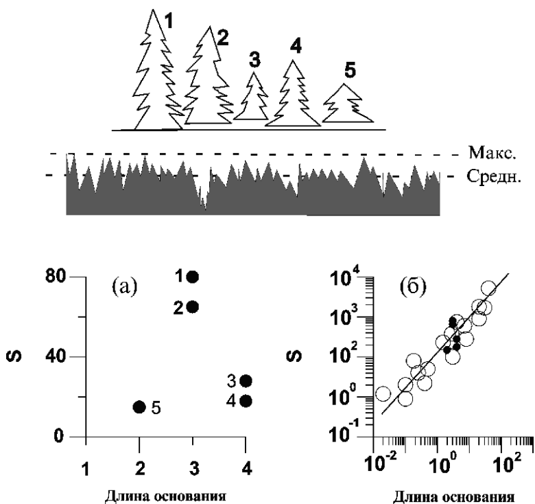
Рис. 2.5. Численный эксперимент. В верхней части рисунка – единичные ели; ниже – еловый лес. (а) – соотношение длины основания ели и площади ( S ) её боковой проекции (группа из пяти елей), (б) – то же самое в составе леса. В условных единицах. Пояснения в тексте.
