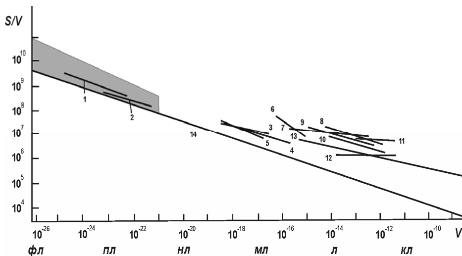
Рис. 7.21. Соотношение удельной поверхности ( S/V , \text{км}^{-1} ) и объёма ( V , \text{км}^3 ) у одноклеточных и многоклеточных водорослей 1, 2 – морские диатомовые; 3 – 5 – осевые структуры первого-третьего порядков цистозииры косматой; 6 – пtilота; 7 – 11 – ламинария сахаристая из разных местообитаний Баренцева моря; 12 – ламинария цикориеподобная из Японского моря; 13 – высшие наземные растения (кустарники, деревья); 4 – соотношение S/V и V у тел сферической формы и многоклеточных водорослей. (по: Хайлов и др., 1992)
