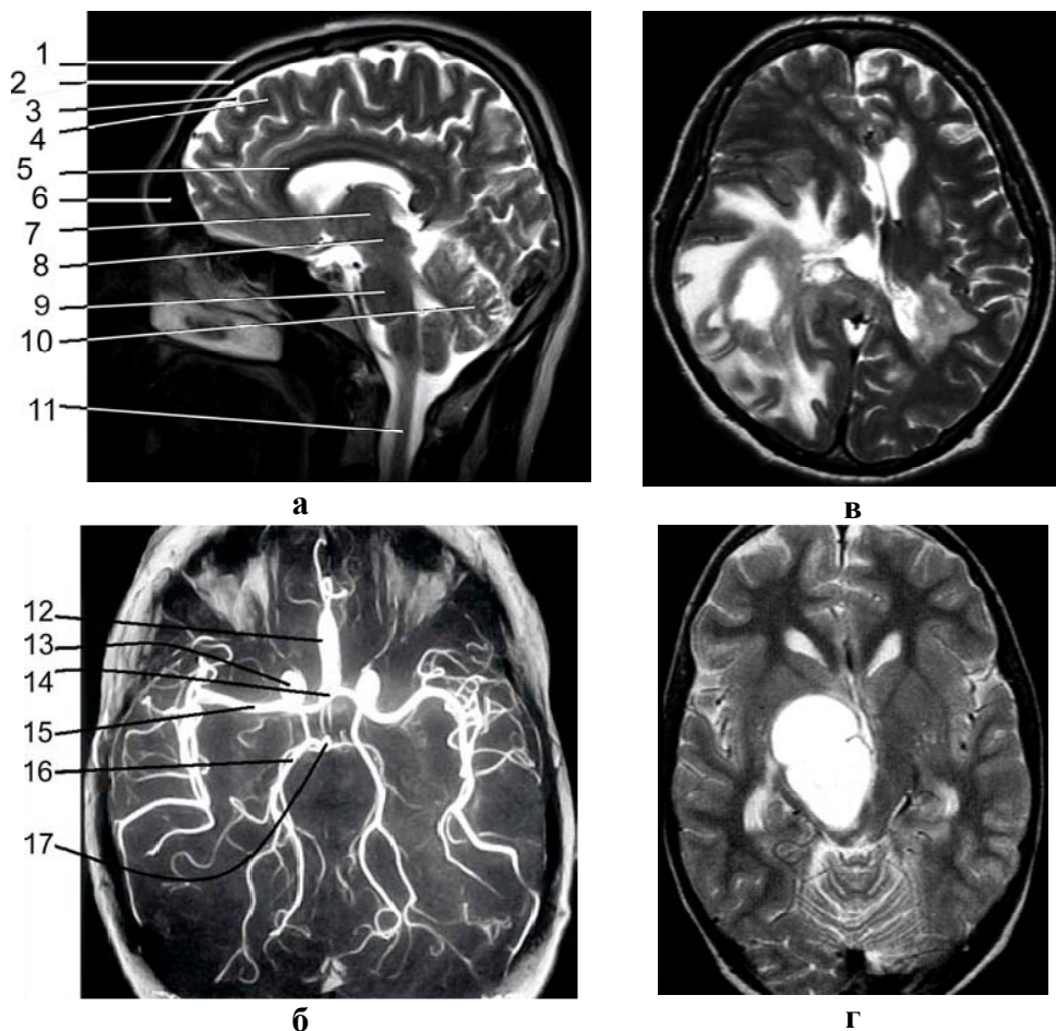
Рис. 6.13. Примеры Мр томограмм:
