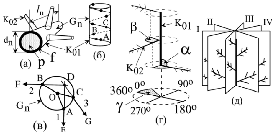
Рис. 5.9. Элементы пространственной организации ветви первого порядка Cystoseira crinita . а – осевая структура первого порядка с осявыми структурами второго порядка и ее поперечное сечение; б – схема основной генетической спирали (Точками указаны места положений осей следующего порядка.); в – д – схемы пространственного расположения осей второго порядка. l_n , d_n – длина и диаметр осевой структуры; ткани, содержащие (f) и не содержащие (p) пигменты; А, В, С - места расположений осевых структур K_{02} под номерами 1, 2 и 3 на оси K_{01} ; \angle AOB , \angle BOC – углы расхождения; \angle EDF и развернутый \angle FDG – углы поворота; \alpha , \beta , \gamma – углы наклона, поворота и азимутальный угол ветвей второго порядка; I, II, III, IV – плоскости радиального сечения ветви первого порядка. Остальные обозначения те же, что на рис. 5.4.
