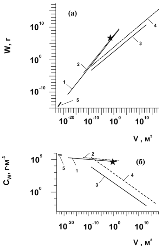
Рис. 9.23. Телесные и надтелесные объекты совмещены здесь по параметрам V и W в общей биосферной метрике.
