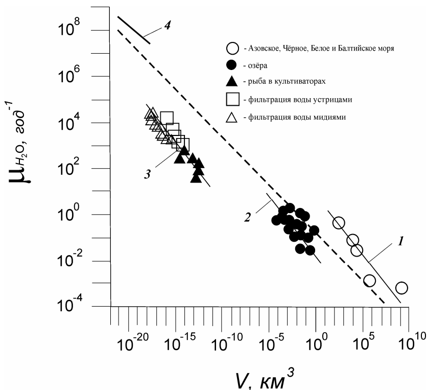
Рис. 8.6. Соотношение между геометрическим объёмом ( V_n, V_{n+1} ) водных биокосных объектов и интенсивностью водообмена ( \mu_{\text{воды}} ) в них. Обозначения: моря: Азовское, Чёрное, Белое, Балтийское (1); рыба в культиваторах (2); фильтрация воды мидиями ( \Delta ) и устрицами ( \square ); движение крови в капиллярных сосудах (4). Штриховая линия – обобщающий тренд.
