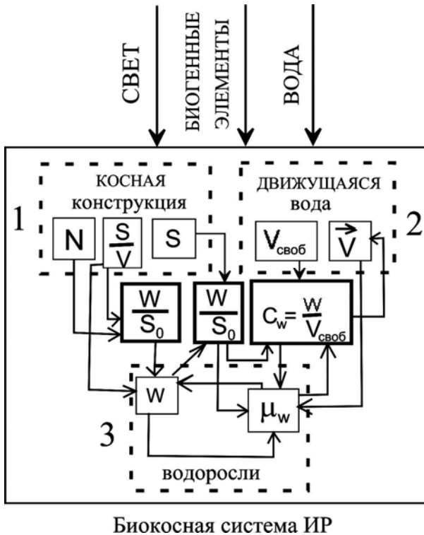
Рис. 6.5. Блок-схема управления фитообращением в составе ИР. Пояснения в тексте.
