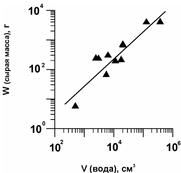
Рис. 4.2. Соотношение объема (V) литоральных ванн и общей массы (W) донных многоклеточных водорослей в них. Баренцево море.
