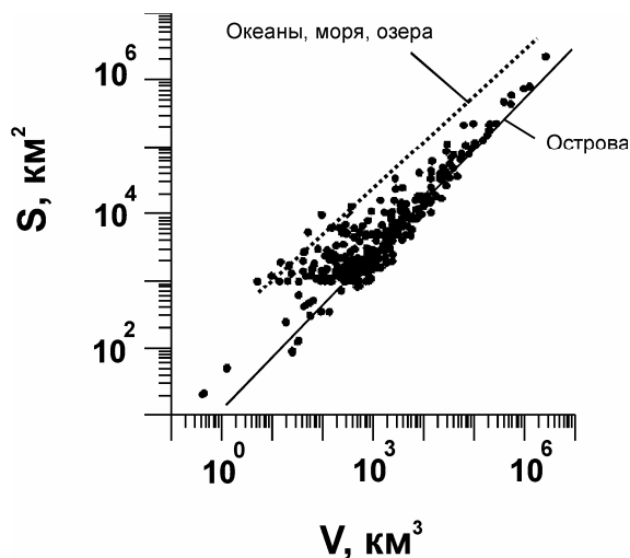
Рис. 4.5. Здесь показано соотношение между индивидуальным объемом V и площадью внешней поверхности S в разменных рядах островов (точки) и тренд сплошной линией) и водоемов (штриховая линия). Как видим, регрессии почти параллельны. (Рисунок взят из книги, названной в подписи к рис.4.4).
