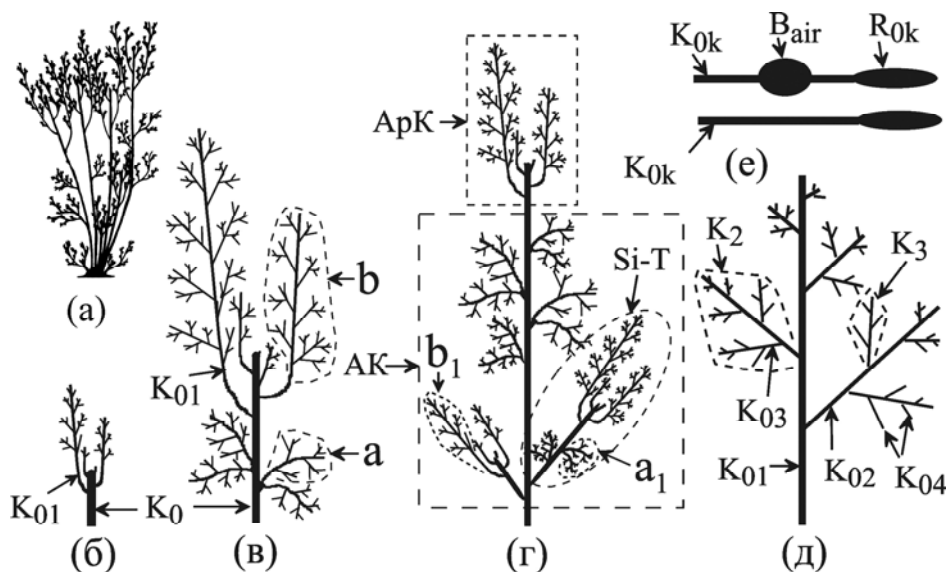
Рис. 5.1. Макроморфо-структурная организация слоевища цистозирры косматой ( Cystoseira crinita (Desf.) Bory):
