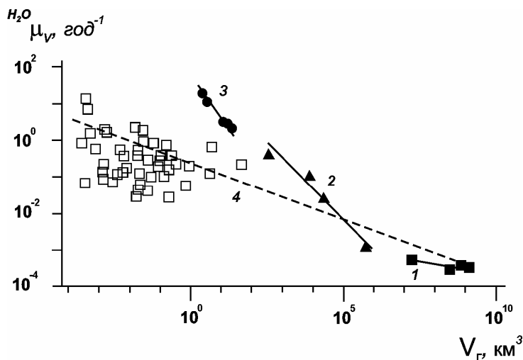
Рис. 9.6. Соотношение геометрического объёма, занимаемого водой ( V_{\text{Г}} ), и интенсивности водообмена ( \mu_{\text{H}_2\text{O}} ) в водоемах разного типа (стационарное состояние): 1 – океаны, 2 – моря, 3 – водохранилища, 4 – озера.
