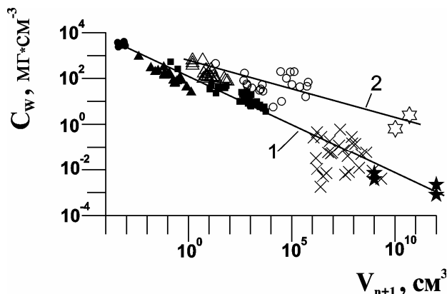
Рис. 3.11. Соотношение объема и объемной концентрации “живого вещества” растений в обитаемых пространствах разных телесных (ткани морской водоросли цистозире ●) и надтелесных (все остальные объекты) фитосистем: ветки цистозире (▲), целые слоевища цистозире (△), полог цистозире на морском дне (■), полог лугового травостоя (○), озера с фитопланктоном (×), сообщества фитопланктона в фотическом слое Черного моря (★), яблони в их кронах (☆).
