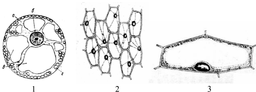
Рис. 8.10. Некоторые варианты формы рстительной клетки. 1– поперечный срез цилиндрической клетки: а – цитоплазма; б – ядро; в – вакуоли; г – хлоропласты. 2, 3 – группа растительных клеток и единичная растительная клетка.
