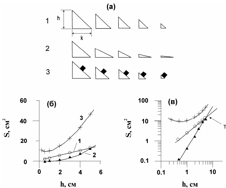
Рис. 2.3. Численный эксперимент. (а) – фигуры идеальной геометрической формы (треугольники). h – высота, k – длина основания, S – площадь поверхности фигуры. (б) – соотношение площади ( S ) указанных выше фигур и их высоты ( h ). (в) – то же соотношение, но в двойных логарифмических координатах. Пояснения в тексте.
