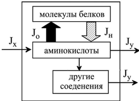
Рис. 7.4. Схема круговорота веществ на молекулярно-клеточном уровне (Азотный обмен). J_o , J_n – синтез и ресинтез молекул белка. Остальные обозначения те же, что на рис. 7.3.
