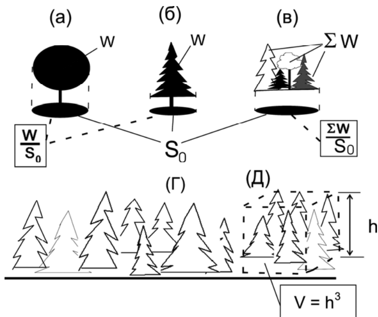
Рис. 3.12. Способы геометрической аппроксимации внешних форм отдельных растений и их совокупностей. Пояснения в тексте.
