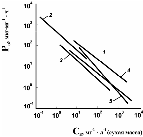
Рис. 3.13. Связь интенсивности гетеротрофного накопления углерода глюкозы с концентрацией живой массы в популяциях отдельных видов морского фитопланктона в условиях культур: 1 – Prorocentrum micans ; 2 – Cymnodinium lanskaya , 3 – Gyrodini sp., 4 – Cymnodinium kovalevskii ; 5 – Cymnodinium foliaceum .
