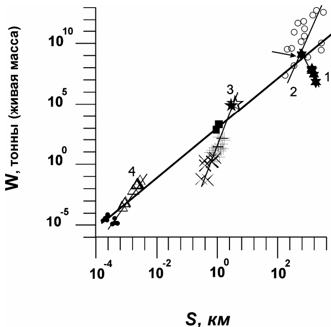
Рис. 4.7. Соотношение площади земной поверхности биокосных фитосистем разного типа ( S_0 ) и общей массы (W) обитающих на ней наземных или водных растений. Линии на рисунке обобщают следующие объекты:
