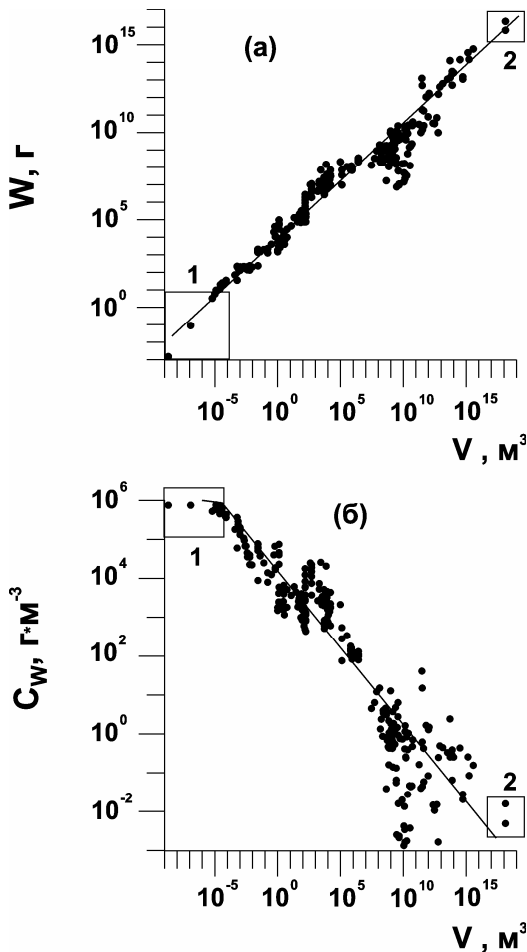
Рис.4.10. Соотношение между объемом ( V ) обитаемого пространства и массой ( W ) живого вещества в них. На рисунке обобщены данные о наземных и водных биокосных системах с животными; использованы данные, показанные на рис. 4.9 и некоторые другие. В диапазоне от 10 - 8 (квадрат 1, долгоносики в стручках люцерны) до 1018 \text{ м}^3 (квадрат 2, зообентос и зоопланктон в Мировом океане) объем обитаемого пространства и живая масса обитателей закономерно связаны между собой. Следствием соотношения между V и W является обратная зависимость между V и C_w , т.е. концентрацией живого вещества обитателей в тех же биокосных системах (рисунок «б»).
