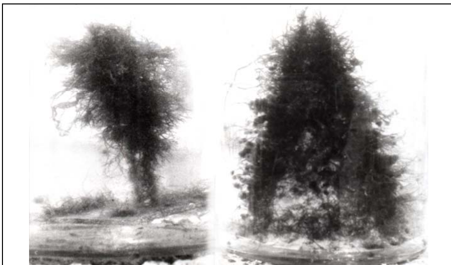
Рис. 6.1. Установленные на подводном стенде и обросшие многоклеточными водорослями стержень (а), конус (б).
