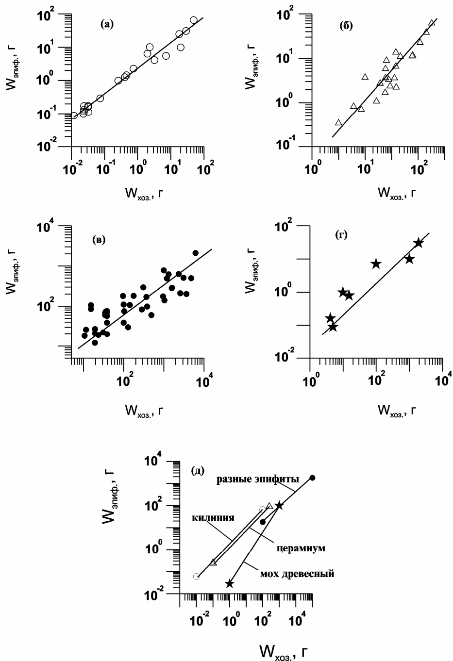
Рис. 4.8. Соотношение общей массы эпифитов ( W_{\text{эпиф}} ) и массы “хозяина” ( W_{\text{хоз}} ). “Хозяином” мелких морских водорослей являются слоевища более крупных водорослей, в данном случае черноморской цистозеры. “Хозяином” древесного мха служат веточки деревьев. а, – килиния на цистозере, б – церамиум на цистозере, в – все эпифиты цистозеры на ее ветвях, г – мох на веточках дерева. На рис. 4.8 д в общей метрике сравниваются все показанные на рис. 4.8 а – г случаи эпифитирования .
