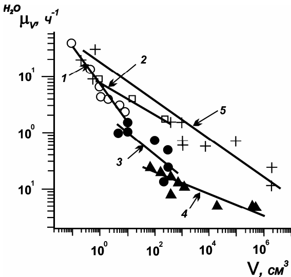
Рис. 9.8. Соотношение стационарного объема воды ( V ) и интенсивности водообмена ( {}^{H_2O}\mu_v ) у водных и наземных животных: 1 – мидии; 2 – морские гребешки; 3 – пресноводные рыбы; куры, собаки, лошади; 4 – в проточных аквакультурных системах.
