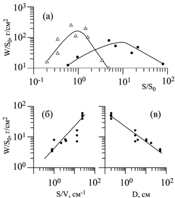
Рис. 6.3. Пример управления биомассой макрофитов на поверхности единичных стержней:
