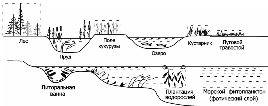
Рис. 3.16. Схема, показывающая ряд наземных и водных биокосных фитосистем. Все они имеют занимаемую ими площадь земной поверхности и общую массу обитающих на ней наземных или водных растений. На рис. 4.2 будет показано соотношение этих величин в размерном ряду таких объектов.
