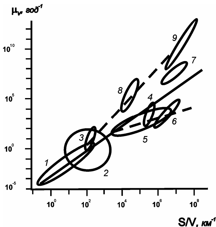
Рис. 9.11. Связь удельной поверхности ( S/V ) и интенсивности водообмена ( {}^{H_2O}\mu_v ) на разных уровнях организации биогидросферы (объекты и обозначения те же, что и на предыдущем рисунке). Сплошная линия проведена по данным о водообмене в океанах, морях, озерах, и экстраполирована в зону S/V организмов, их органов и тканей. Верхняя штриховая линия обобщает водообмен крови в органах человека и кровеносных сосудах, нижняя штриховая линия обобщает водообмен в телах животных и растений.
