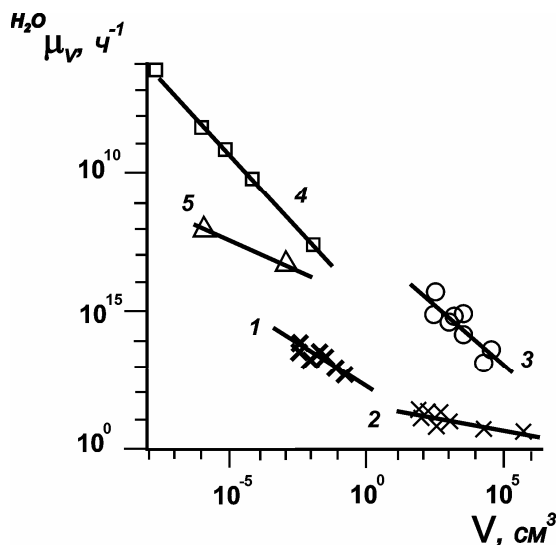
Рис. 9.9. Соотношение стационарного объема воды ( V ) и интенсивности водообмена ( {}^{\text{H}_2\text{O}}\mu_V ) в тканях морской водоросли аларии (1), в телах наземных животных (2), в кровоснабжаемых органах человека (3) и в кровеносных сосудах мозга собаки (4). Для сравнения регрессия 5 показывает объемную интенсивность фильтрационного водообмена у морского зоопланктона
