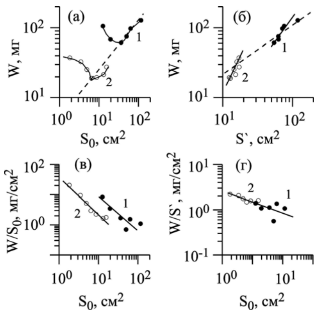
Рис. 6.10. а, б – Соотношение между биомассой водорослей на конусах W и геометрическими характеристиками конусов – S'/S_0 и S' ; в, г – Соотношение между параметрами обрастания конусов ( W/S_0 и W/S' ) и площадью поверхности их дна ( S_0 ) при их одинаковом телесном объеме конусов. Обозначения: серия 1Д – черные кружки, серия 2Д – светлые кружки. См. текст.
