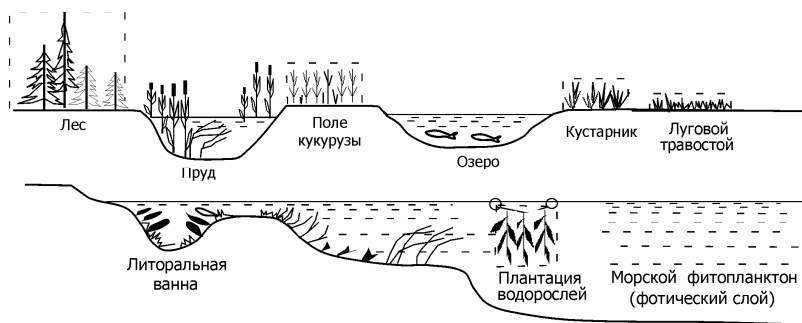
Рис. 9.15. Схема, показывающая ряд наземных и водных биокосных фитосистем. Все они имеют занимаемую ими площадь земной поверхности и общую массу обитающих на ней наземных или водных растений.
