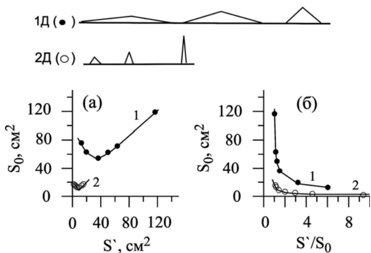
Рис. 6.9. Соотношение двух базовых параметров обитания – S'/S_0 и S_0 . Соотношение S'/S_0 отражает геометрический смысл понятий - “уплощенные”, “распластанные” конусы (серия 1Д, в верхней части рисунка) и “вытянутые”, “вздымающиеся” конусы (серия 2Д). Кривые на графике показывают, как в ряду конусов изменяется содержащаяся в них “геоморфологическая информация”, передаваемая затем в поселившиеся на конусах сообщества водорослей.
