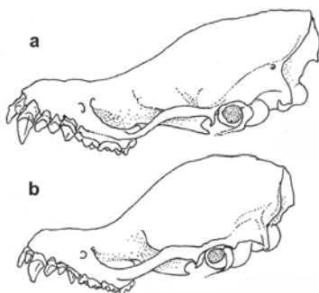
Fig. 31. Skull profiles of Kerivoula : a) K. kachinensis ; b) K. titania .
