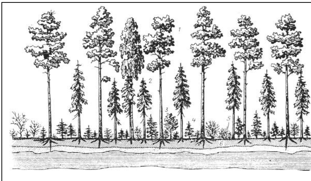
Рис. 7. Компоненты леса:
