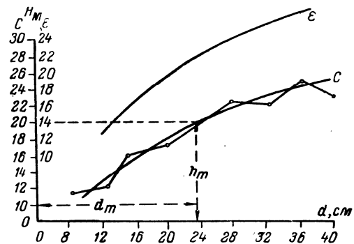
Рис. 136. Графики высот
