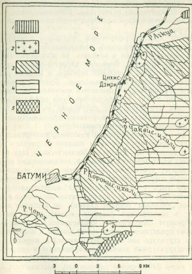
Рис. 1. Схематическая геолого-петрографическая карта окрестностей Батуми.
