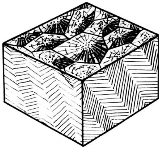
Рис. 38. Блок-диаграмма конусной структуры (по: Попов, 1992, рис. III)
