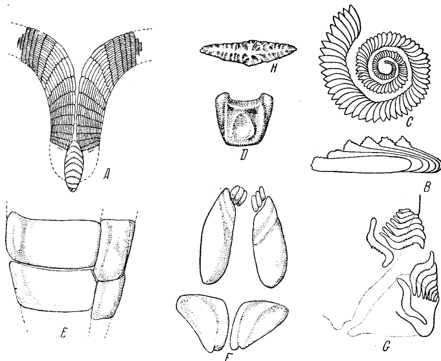
Рис. 33. Зубы брахиодонтов:
