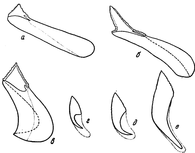
Рис. 24. Зубные сегменты:
