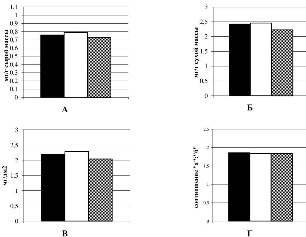
Рис. 34. Содержание хлорофилла (а+б) в листьях залежных растений на разных стадиях дему- тации: А – мг/г сырой массы, Б – мг/г сухой массы, В – мг/дм 2 , Г – соотношение «а» + «б». Условные обозначения: ■ – бурьянистая стадия, □ – корневищная стадия, ▨ – рыхлокустовая стадия
