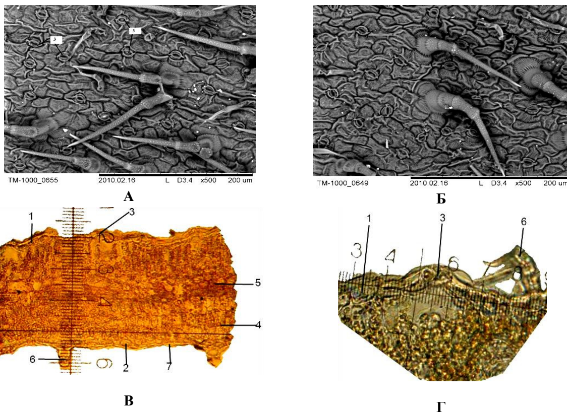
Рис. 32. Анатомическая структура листа Heteropappus altaicus (Willd.) Novopokr. Условные обозначения: А – бурьянистая (16x20), Б – рыхлокустовая стадии (20x40): 1 – верхний эпидермис, 2 – нижний эпидермис, 3 – устьице, 4 - столбчатая ткань, 5 – губчатая ткань, 6-волоски, 7 - кутикула
