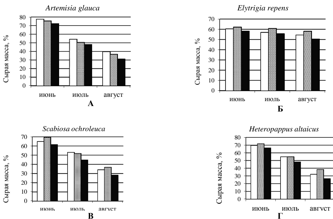
Рис. 33. Содержание общей воды в листьях растений по стадиям восстановления (%) 2009 г.: А – Artemisiaglauca , Б – Elytrigiarepens , В – Scabiosaochroleuca , Г – Heteropappusaltaicus . Условные обозначения: □ – бурьянистая, ▨ - корневищная, ■ – рыхлокустовая стадии
