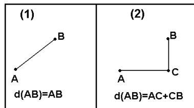
Рис. 41. Эвклидово (1) и манхэттенское (2) расстояния
