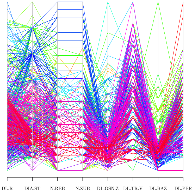
Рис. 36. График параллельных координат
