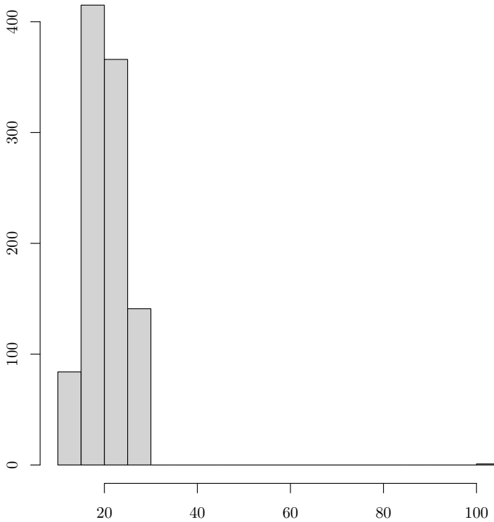
Рис. 11. Гистограмма зарплат 1007 гипотетических сотрудников
