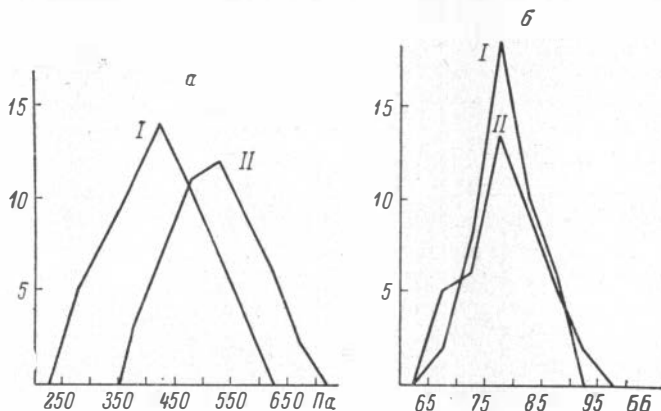
Рис. 23. Изменчивость ростров Passaloteuthis tolli (Pavl.) (I) и Passaloteuthis viluensis Krimh. (II).
