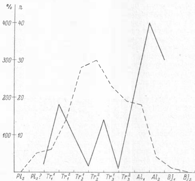
Рис. 60. Колебания количества видов (пунктир) и коэффициента изменения видового состава (сплошная линия) сибирских Nannobelinae , Passaloteuthinae и Hastitidae в ранней юре и первой половине средней юры.
