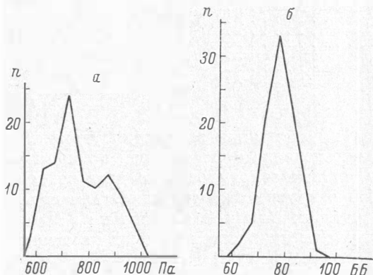
Рис. 31. Изменчивость ростров Catateuthis subinaudita (Voron.).
