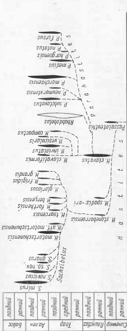
Рис. 55. Схема предполагаемого развития видов сем. Hastitidae .
