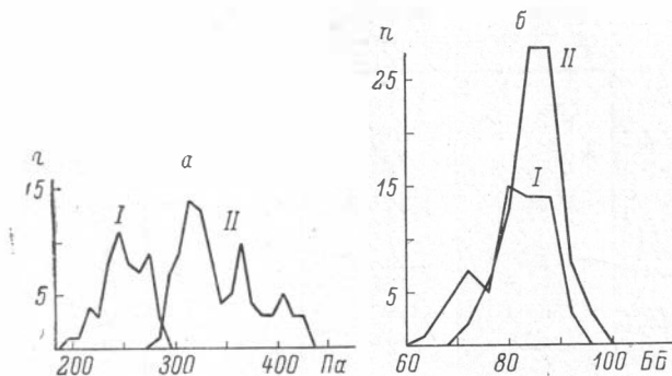
Рис. 16. Изменчивость ростров Brachybelus (Brachybelus) dagysi Sachs sp. nov. (I) и B. (B.) kirinae Sachs sp. nov. (II).
