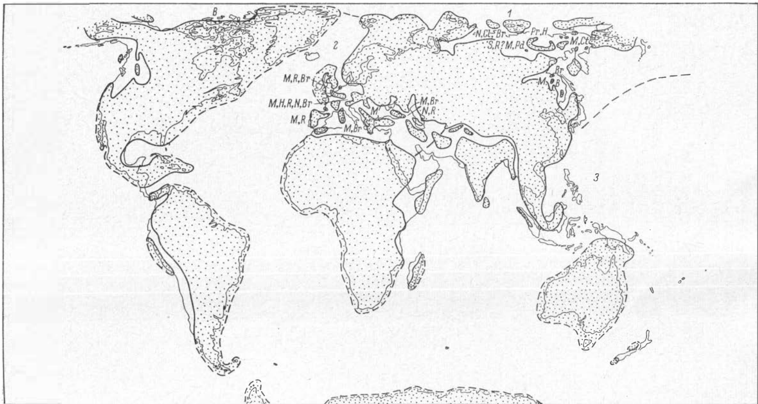
Рис. 62. Схема географического распространения белемнитов в раннеэоценовое время. Условные обозначения см. под рис. 56.
