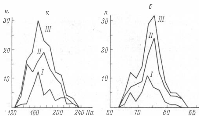
Рис. 5. Изменчивость ростров Nannobelus krimholzi Sachs sp. nov.
