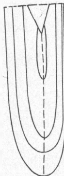
Рис. 34. Продольное сечение ростра Dactylotheuthis aff. irregularis (Schlotheim), № 85-222, верхний тоар, бассейн р. Вилюя.
