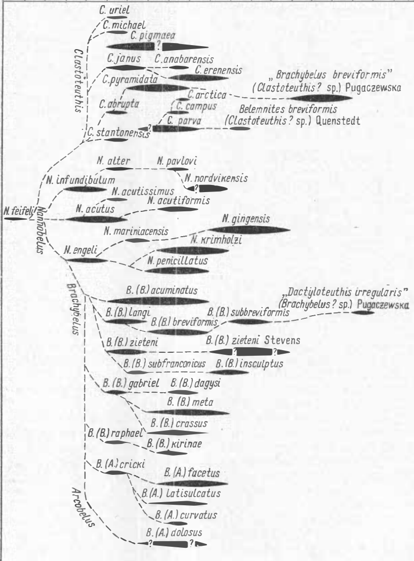
Рис. 53. Схема предполагаемого развития видов подсемейства Nautiloidea .
