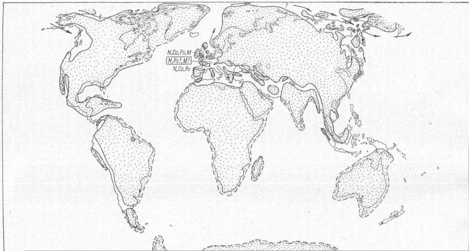
Рис. 56. Схема географического распространения белемнитов в геттанг-синемюрское время.
