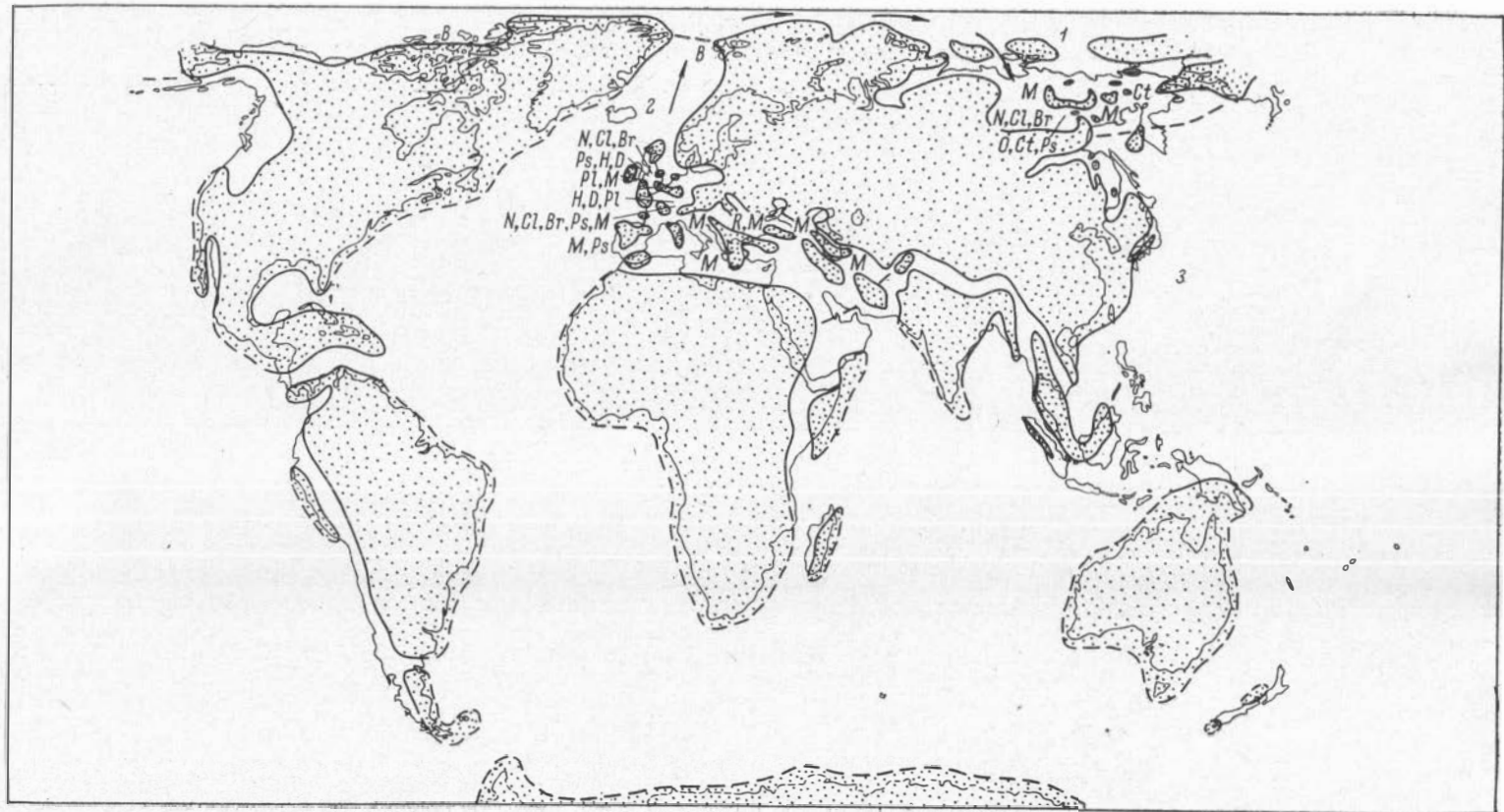
Рис. 58. Схема географического распространения белемнитов в раннеюрское время.
