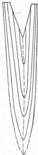
Рис. 38. Продольное сечение ростра Orthobelus obscurus Naln. sp. nov., № 85-236, средний—верхний тоар, р. Келимээр, бассейн р. Оленек. ×0.6.
