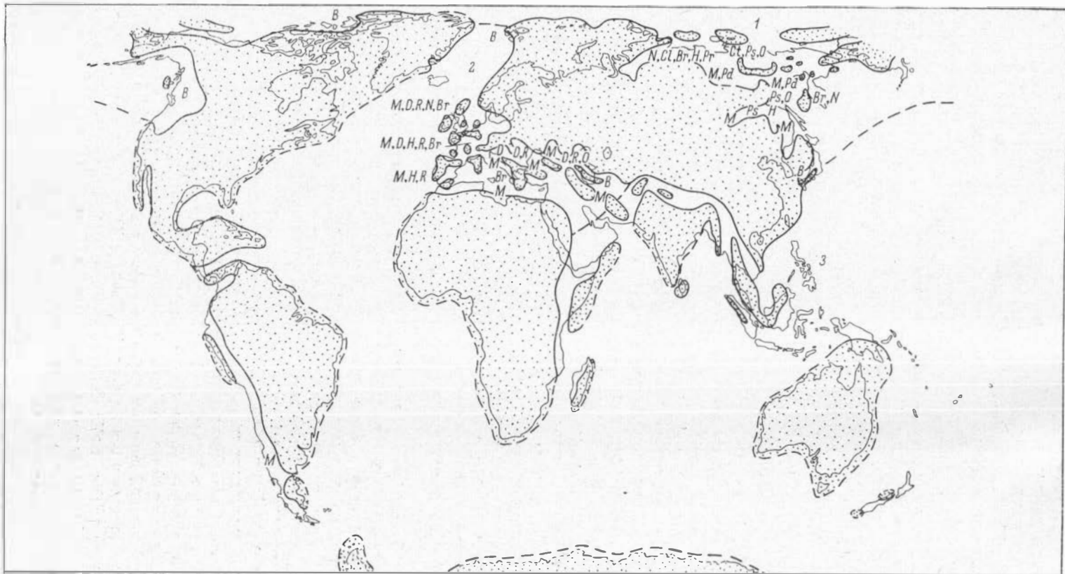
Рис. 61. Схема географического распространения белемнитов в позднегоарское время.
