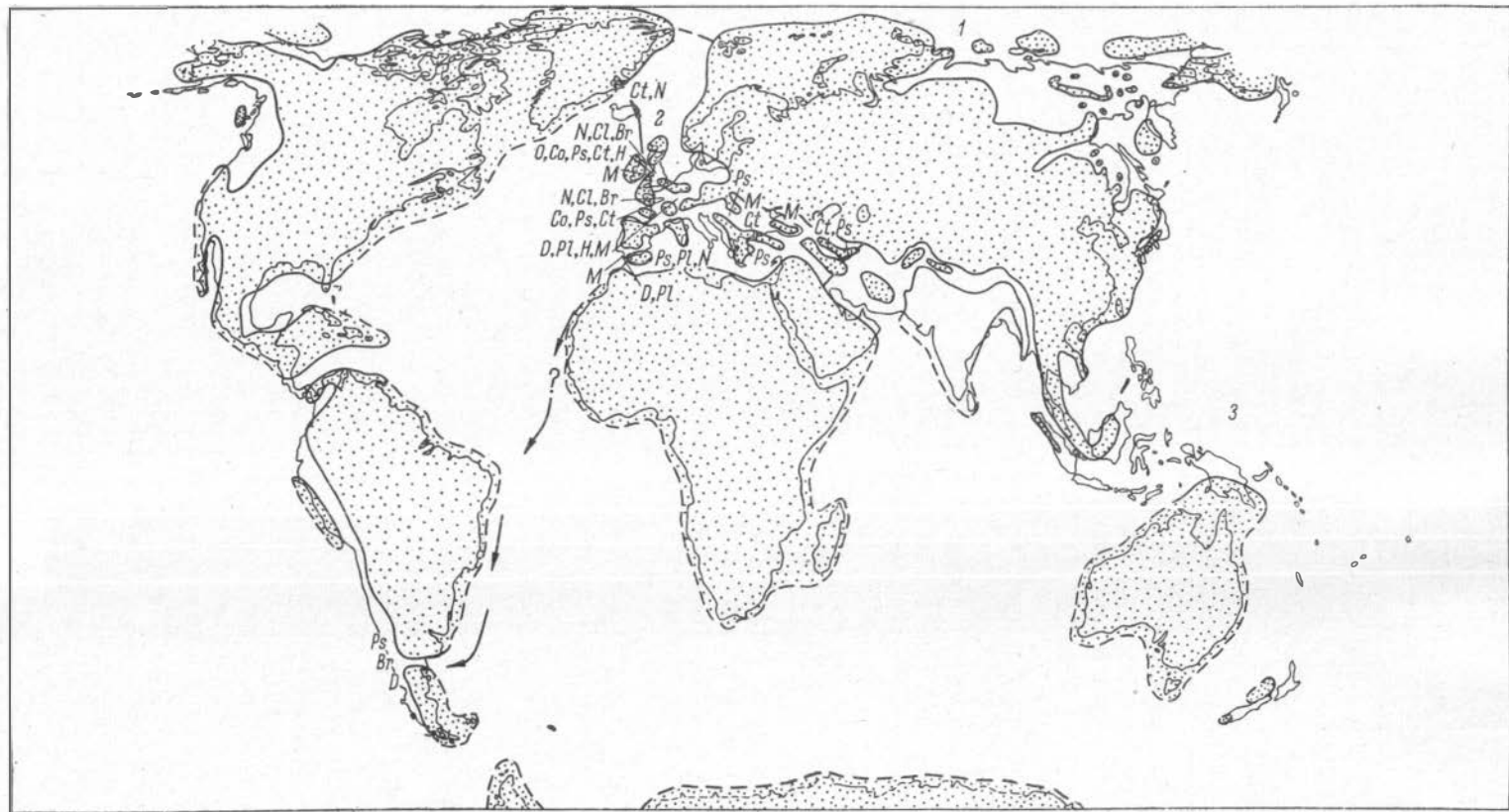
Рис. 57. Схема географического распространения белемнитов в плисбахском веке.
