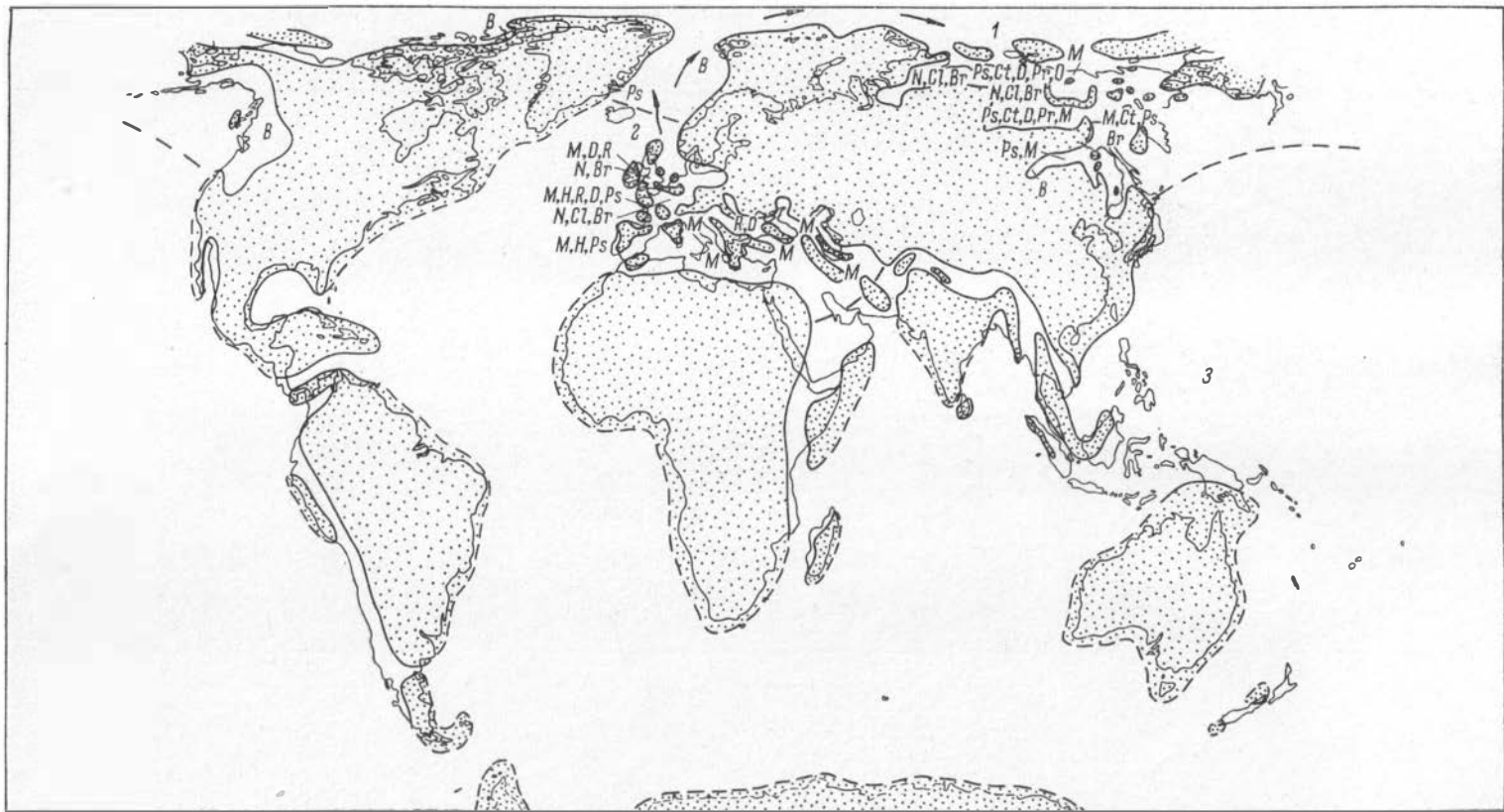
Рис. 59. Схема географического распространения белемнитов в среднетоарское время.
