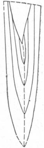
Рис. 39. Продольное сечение ростра Orthobelus gigantoides (Pavl.), № 85-203, средний тоар, зона Dactyloceras commune , побережье Анабарской губы, пачка 4. \times 0.7 .
