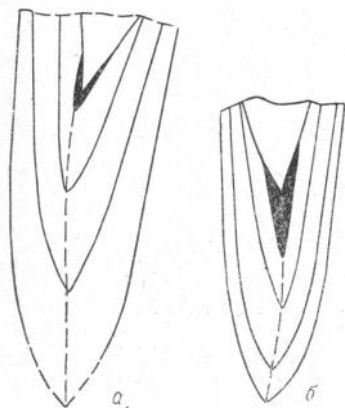
Рис. 4. Продольные сечения ростров Nannobelus krimholzi Sachs sp. nov.
