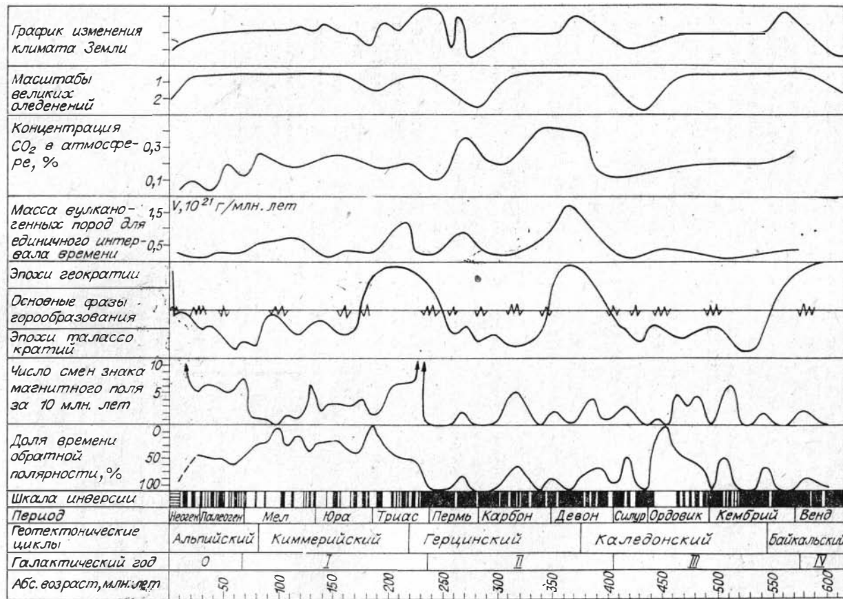
Рис. 10. Динамика геосферы в фанерозое [по Будыко, 1977, 1980; Войлошникову, 1979; Кунину, Сардонникову, 1974].
