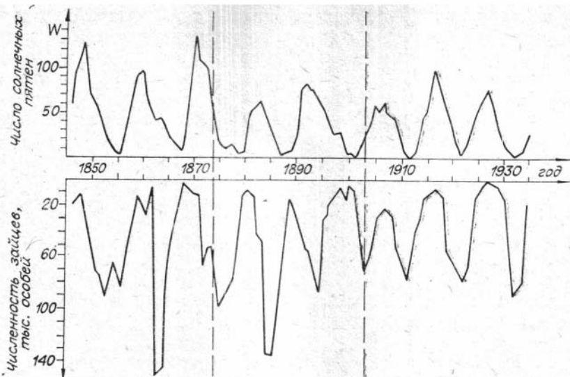
Рис. 8. Динамика изменения численности зайца-беляка в сравнении с числами Вольфа.
