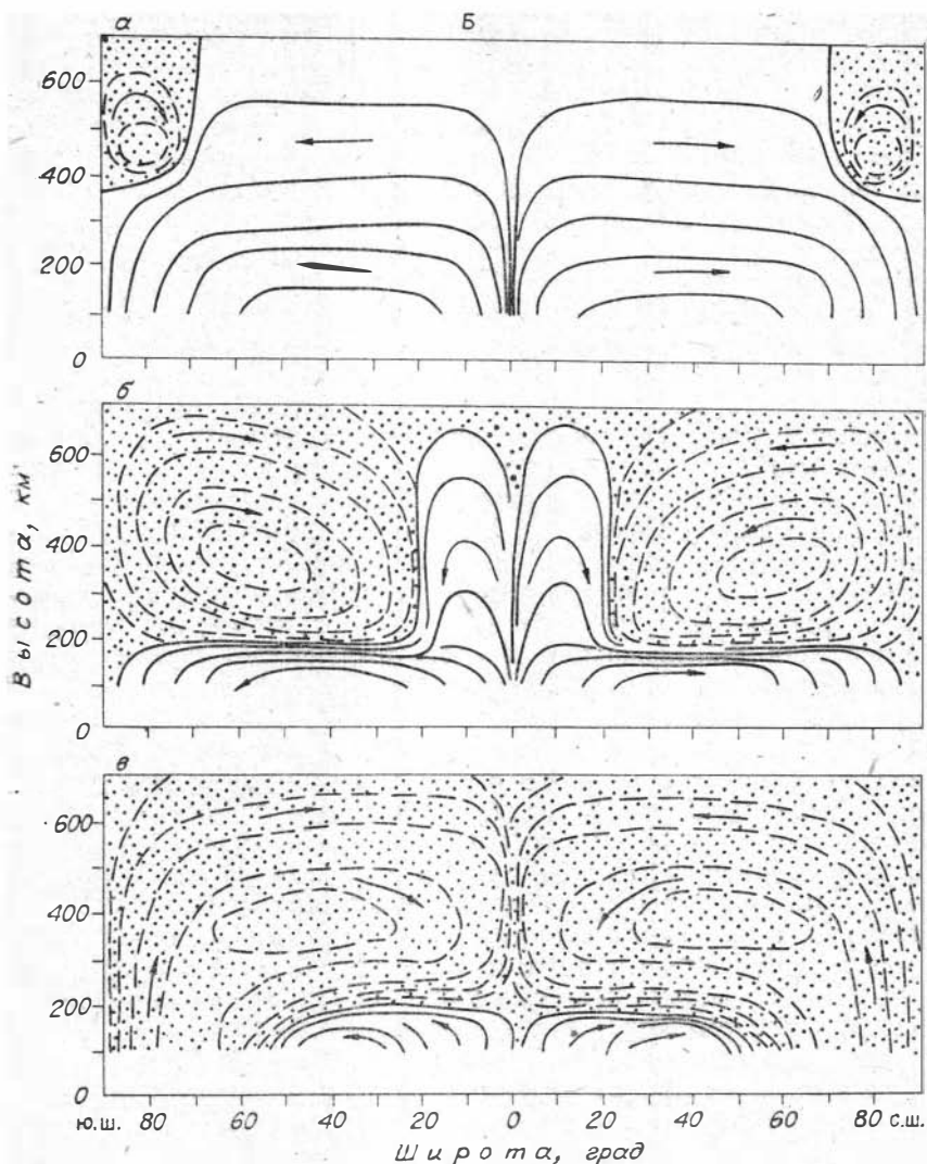
солнцестояния (А) и равноденствия (Б). возмущение; в — магнитная буря.
