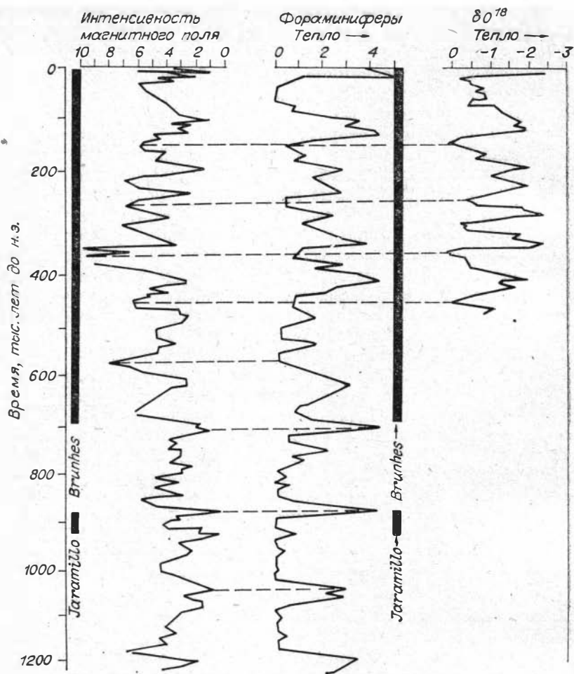
Рис. 6. Изменение температуры океана и напряженности магнитного поля [Wollin, e. a., 1971].
