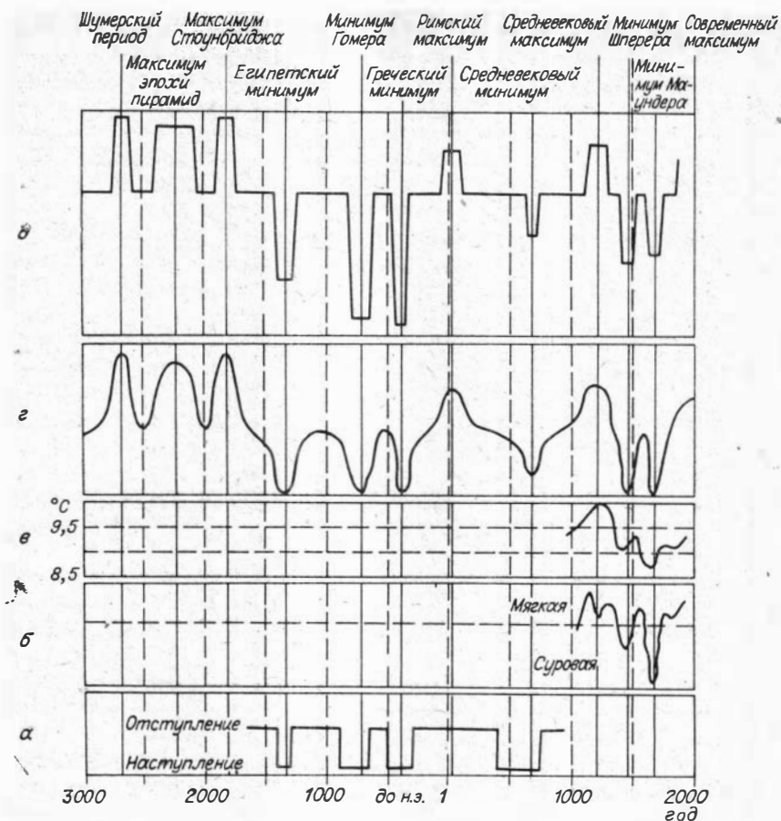
Рис. 4. Реконструкция хода солнечной активности за последние 5 тыс. лет [по Эдди, 1978].
