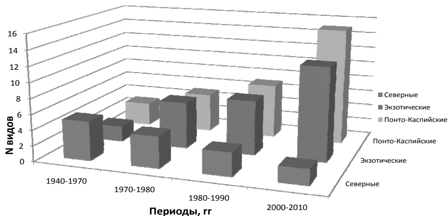
Рис. 2.8. Динамика расселения новых видов рыб в бассейне Волги за период 1940-2010 гг.
