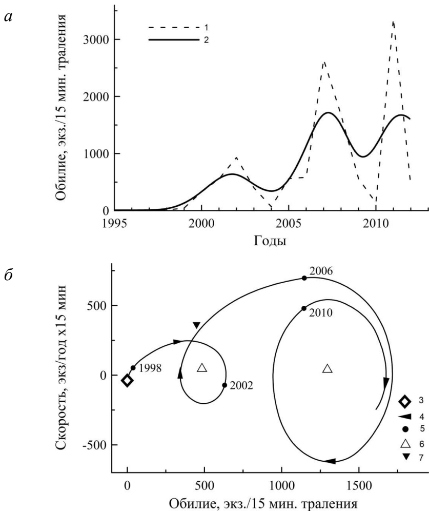
Рис. 7.6. Динамика обилия тюльки (а) и динамический фазовый портрет ее уловов (б) в Рыбинском водохранилище.
