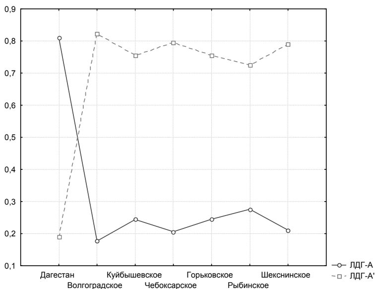
Рис. 8.5. Географическая изменчивость частот аллелей локуса LDH в популяциях тюльки Северного Каспия (Дагестан) и Волжских водохранилищ.
