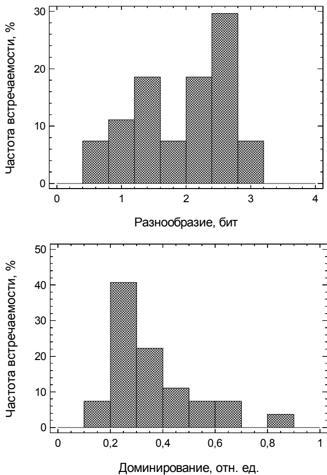
Рис. 5.17. Стационарные (равновесные) уровни разнообразия (а) и доминирования (б) рыбного населения водохранилищ (По: Терещенко, 2000)
