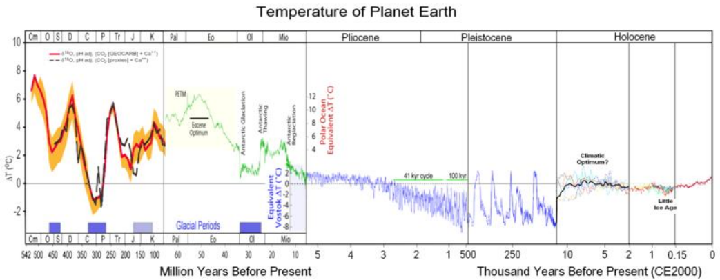
Рис. 1.4. Долговременные температурные колебания (из http://www.wrsc.org/sites/default/files/images/2012/a-2.earth_temperature_record.png ).
