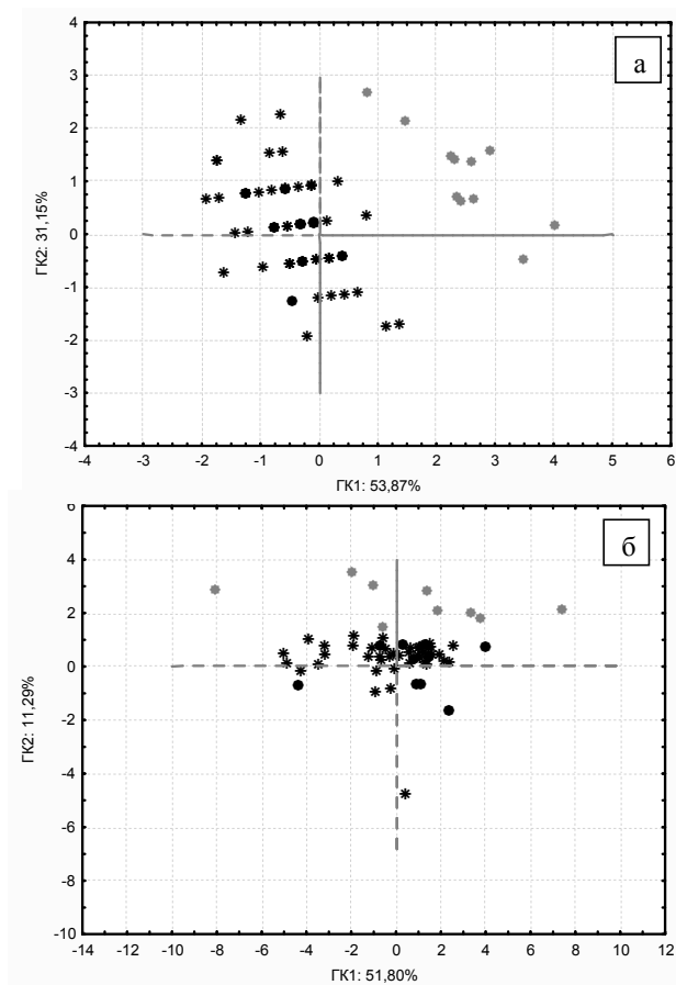
Рис. 8.19. Распределение особей солнечного окуня в пространстве главных компонент по совокупности 4 пластических признаков тела (а) и 9 пластических признаков черепа (б). Условные обозначения: ●- Днепровское водохранилище, * - Дунайский лиман (оз. Ялуг); ●- Днестровский лиман.
