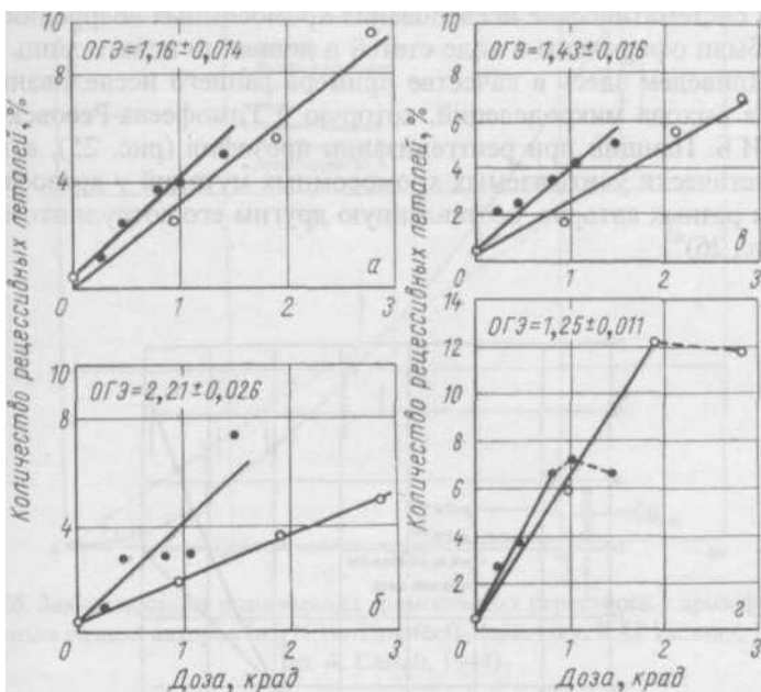
Рис. 24. Кривые доза - эффект для CIB -леталей, индуцированных рентгеновскими лучами \lambda_{эфф} = 0,26 \text{ \AA} (○) и Li + D нейтронами (●).
