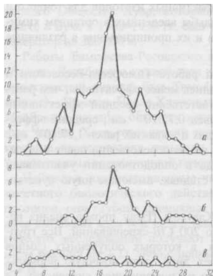
Рис. 23. Распределение выборок (по 200 C1B P_2 культур в каждой) с разным числом мутаций у Drosophila melanogaster после облучения P \text{♂♂} дозой 3000 p.
