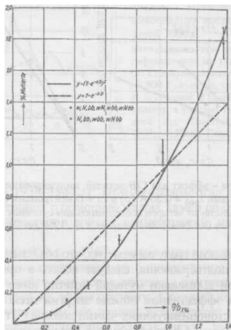
Рис. 25. Кривая доза - эффект для мелких перестроек, вызванных рентгенизацией (делечии с незначительным расстоянием между двумя разрывами) у Drosophila melanogaster (из: N.W. Timoféeff-Ressovsky, K.G. Zimmer, 1947; no: I.B. Panschin, 1946)
