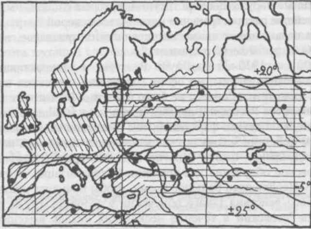
Рис. 12. Относительная жизнеспособность Drosophila funebris из различных регионов Западной Палеарктики:
