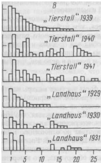
Рис 14. Содержание мутаций в различных свободноживущих популяциях Drosophila funebris (По неопубликованным данным Е.А. и Н.В. Тимофеевых-Ресовских; из: Н. Bauer u. N.W. Timoféeff-Ressovsky, 1943)
