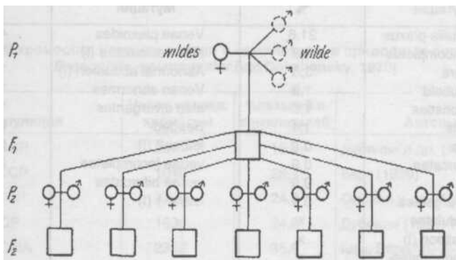
Рис. 4. Схема анализа диких самок, оплодотворенных в природе (по: Н.А. и N.W. Timoféeff-Ressovsky, 1927)
