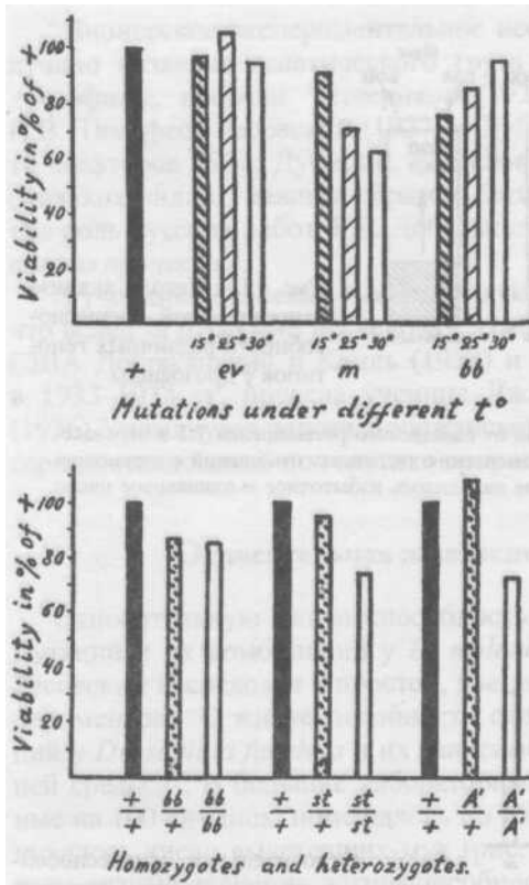
Рис. 7. Относительная жизнеспособность трех мутаций при различной температуре (вверху): отношение частоты вылета мух к частоте вылета нормальных мух при t = 15, 25 и 30^{\circ}\text{C} и постоянном перенаселении культур; и трех мутаций в гетеро- и гомозиготном состоянии (внизу) у Drosophila funebris (По: Тимофеев-Рессовский, 1934.)
