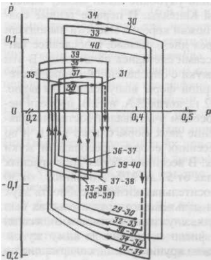
Рис. 15. Адаптационный полиморфизм адалий. Изменения частоты гена A в зимние и летние периоды за 1929-1940 гг. (по: Тимофеев-Ресовский, Свиричев, 1966)
