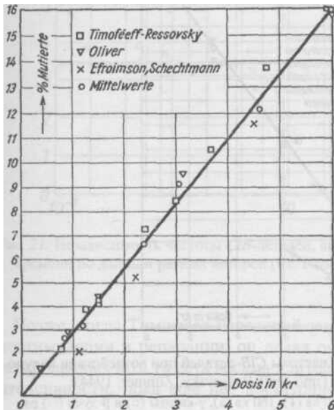
Рис. 19. Зависимость частоты сцепленных с полом мутаций у дрозофил от дозы X-лучей (из: Timoféeff-Ressovsky, 1935): а - результаты опытов Тимофеева-Рессовского; б - сопоставление результатов разных авторов
