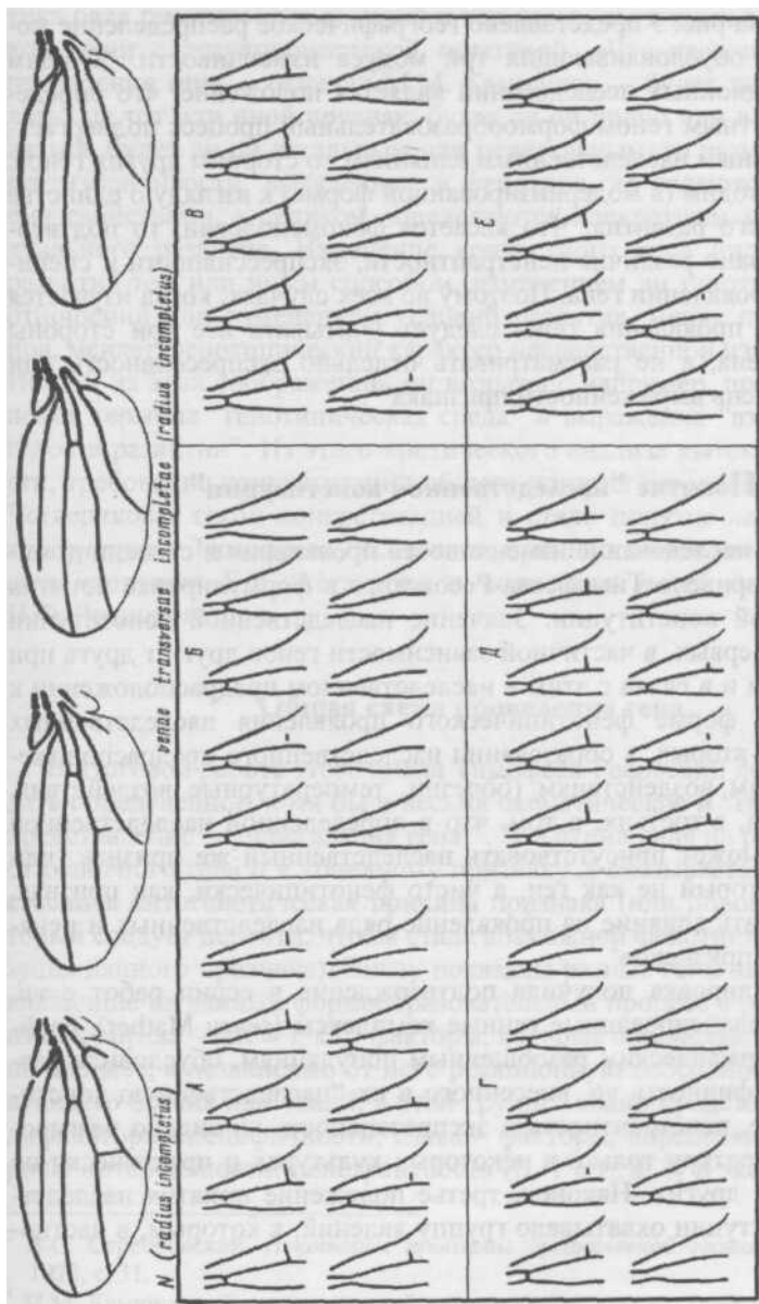
Рис. 1. Влияние генотипической среды на пенетрантность, экспрессивность, специфичность (по: Тимофеев-Рессовский, 1934). A — пенетрантность 100%, экспрессивность слабая, специфичность 1а; B — пенетрантность 100%, экспрессивность сильная, специфичность 1а; B — пенетрантность 60%, экспрессивность сильная, специфичность 1а; Г — пенетрантность 100%, экспрессивность сильная, специфичность 1а; Д — пенетрантность 100%, экспрессивность слабая, специфичность 1а; Е — пенетрантность 100%, экспрессивность слабая, специфичность 1б.
