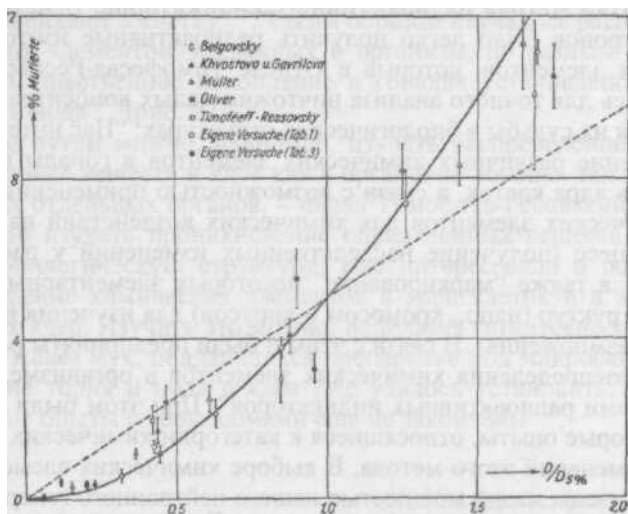
Рис. 26. Зависимость от дозы выхода хромосомных перестроек у дрозофилы по данным разных авторов (из: N.W. Timoféeff-Ressovsky, K.G. Zimmer, 1947; по: A. Catsch, 1944)
