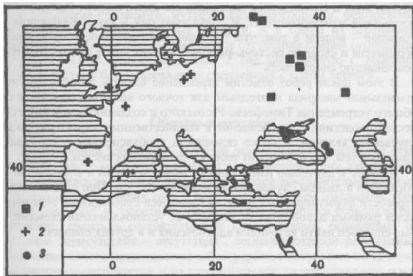
Рис. 3. Географическое распределение генов-модификаторов, определяющих три модуса исчезновения второй поперечной жилки у линии v_1 (по Timoféeff-Ressovsky, 1934a):
