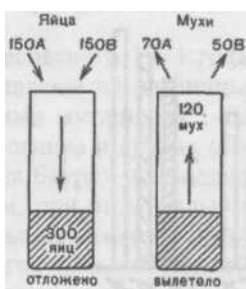
Рис. 5. Метод анализа относительной жизнеспособности различных генотипов у дрозофилы
