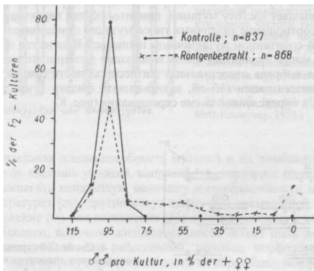
Рис. 9. Вызывание X-лучами мутаций жизнеспособности.
