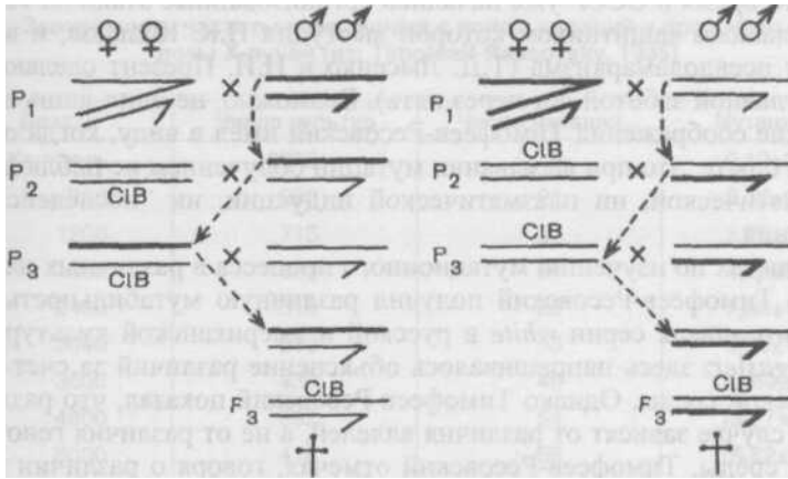
Рис. 18. Схемы скрещивания: а) для выяснения "последствия" облучения, б) для выяснения влияния плазмы (по: Timoféeff-Ressovsky, 1931)
