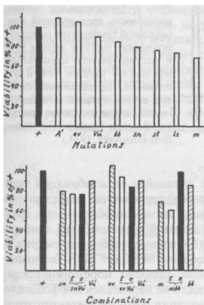
Рис.6. Относительная жизнеспособность восьми различных мутаций (вверху) и трех различных комбинаций этих же мутаций по две (внизу) у Drosophila funebris (частота вылета мух при t = 25^{\circ}\text{C} и среднем перенаселении культур, выраженная в % к частоте вылета нормальных мух)
