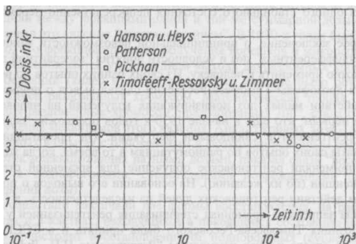
Рис. 21. Независимость частоты CIB -леталей, вызванных облучением, от фактора времени по данным разных авторов (из: Timoféeff-Ressovsky, Zimmer, 1944)
