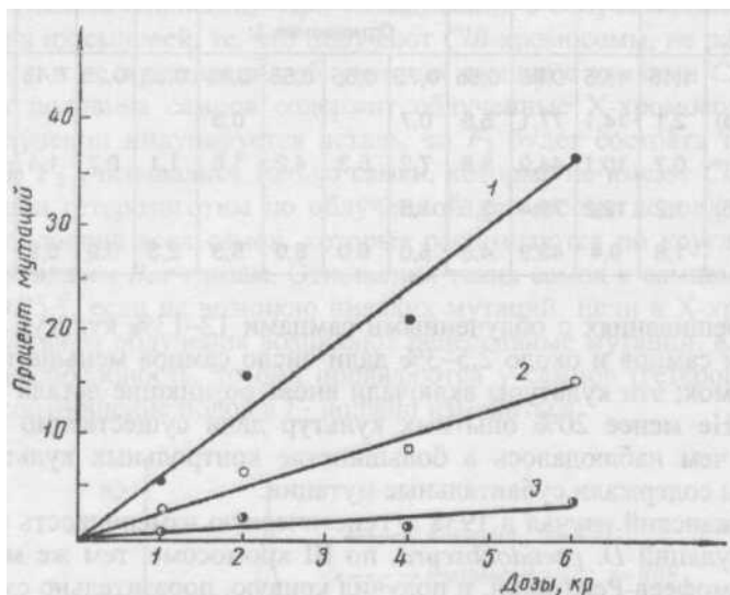
Рис. 10. Кривые эффект - доза сцепленных с полом мутаций у дрозофилы: 1 - понижающих относительную жизнеспособность; 2 - леталей; 3 - сублеталей (по: Тимофеев-Ресовский, 1965)
