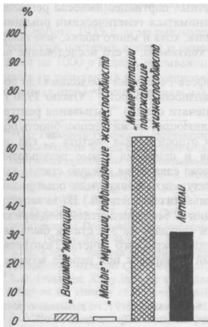
Рис. 11. Соотношение леталей, малых мутаций, понижающих жизнеспособность, малых мутаций, повышающих жизнеспособность и больших мутаций, понижающих жизнеспособность (из: Фонд TP, 45)
