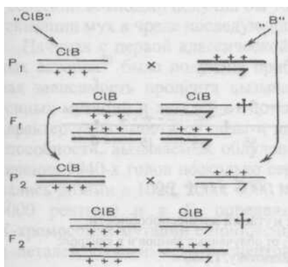
Рис. 8. Схема СШ-скрещиваний для определения относительной жизнеспособности самцов 2-го поколения. Облученные X-хромосомы обозначены жирной чертой (По: Timoféeff-Ressovsky, 1935.)
