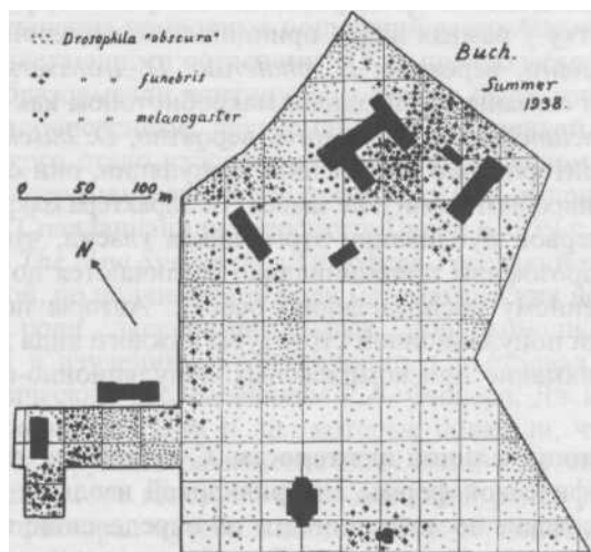
Рис 16. Распределение трех видов Drosophila на участке в Бухе.
