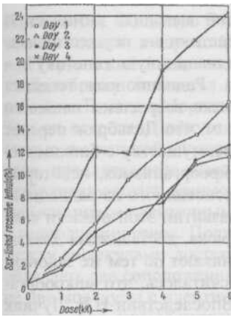
Рис. 28. Кривые доза-эффект для леталей, вызванных на стадиях с разной чувствительностью (из: Zimmer, 1966; по: Traut, 1963)
