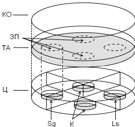
Рис. 1. Схема устройства четырехкамерного ольфактометра: ЗП – запаховые поля; КО – крышка ольфактометра; ТА – тестовая арена; Ц – цилиндр с четырьмя секторами; Sg – чашка Петри с пробой S. granarius ; Ls – чашка Петри с пробой L. serricorne ; К – пустые чашки Петри (контроль).
