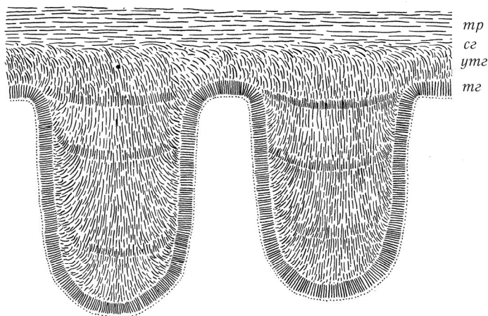
Илл. 39. Схематическое изображение направления роста гиф в базидиуме Thelephora : tr — трама, cg — субгимений, utg — утолщенный гимений, tg — текущий гимений (по: Corner, 1968).
